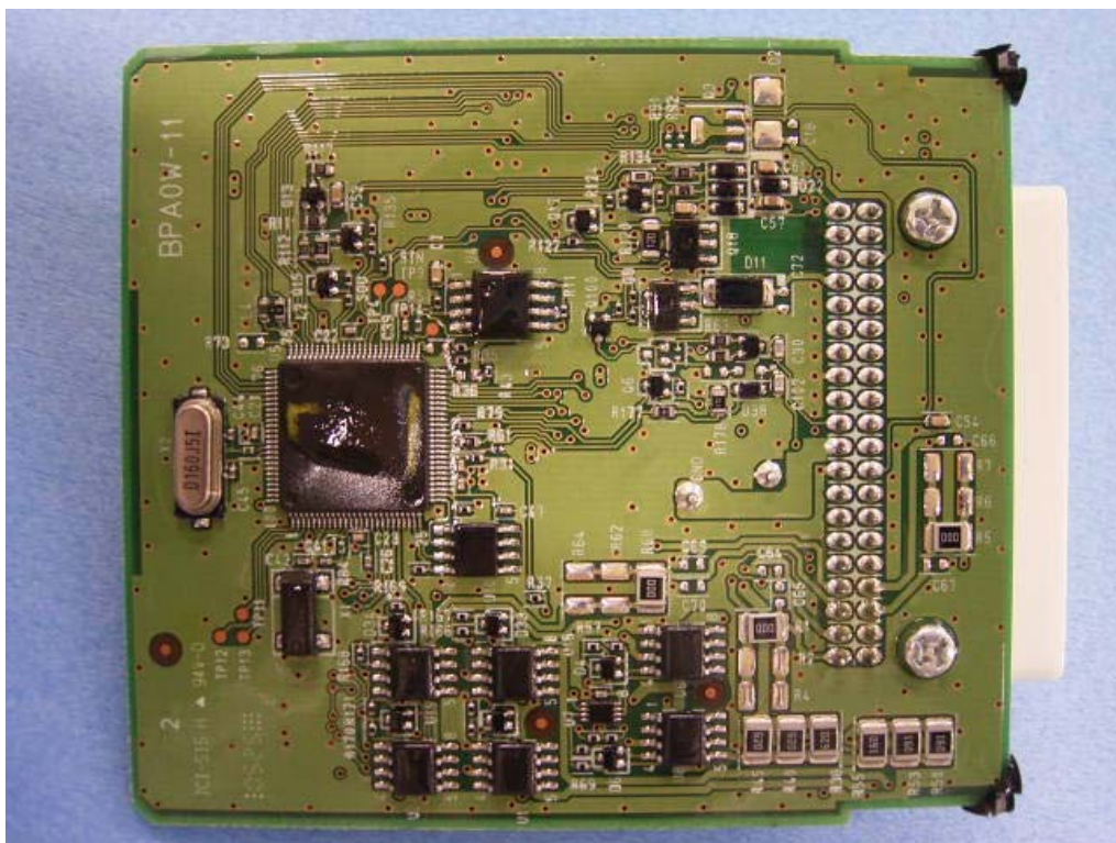
PCB Bottom
