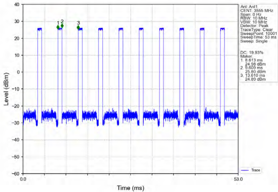
n48_30kHz_SISO_NTNV_10MHz_DFT-s-OFDM QPSK_3555MHz_Inner_Full_Ant1
