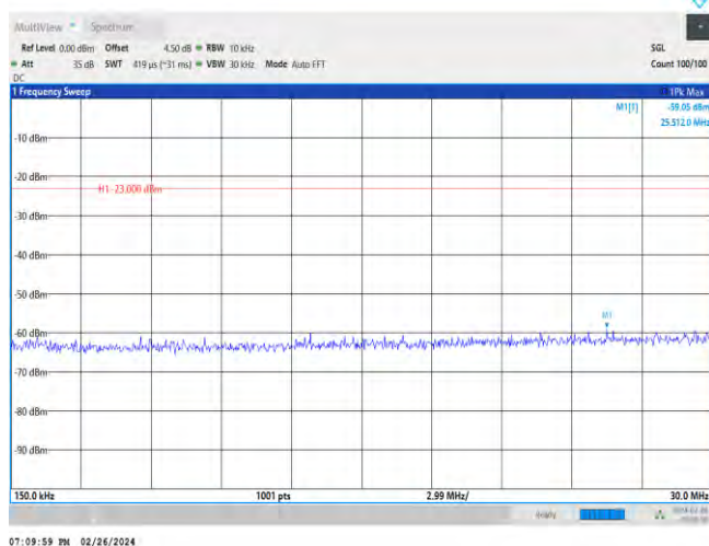
Band26-10MHz-QPSK-26740-1RB#0-Range2:0.15~30MHz
