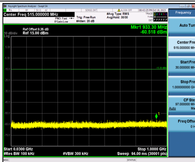
11B_Ant1_2437_30~1000
