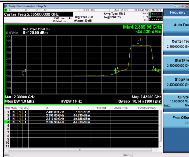
11N20SISO_Ant1_Low_2412_AV
