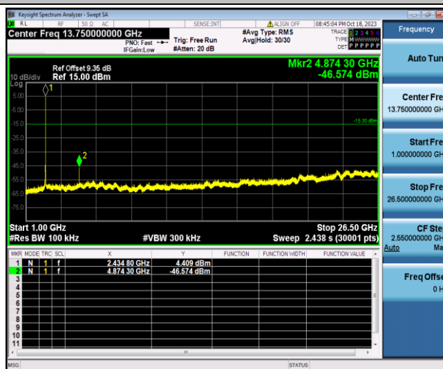
11B_Ant1_2437_1000~26500
