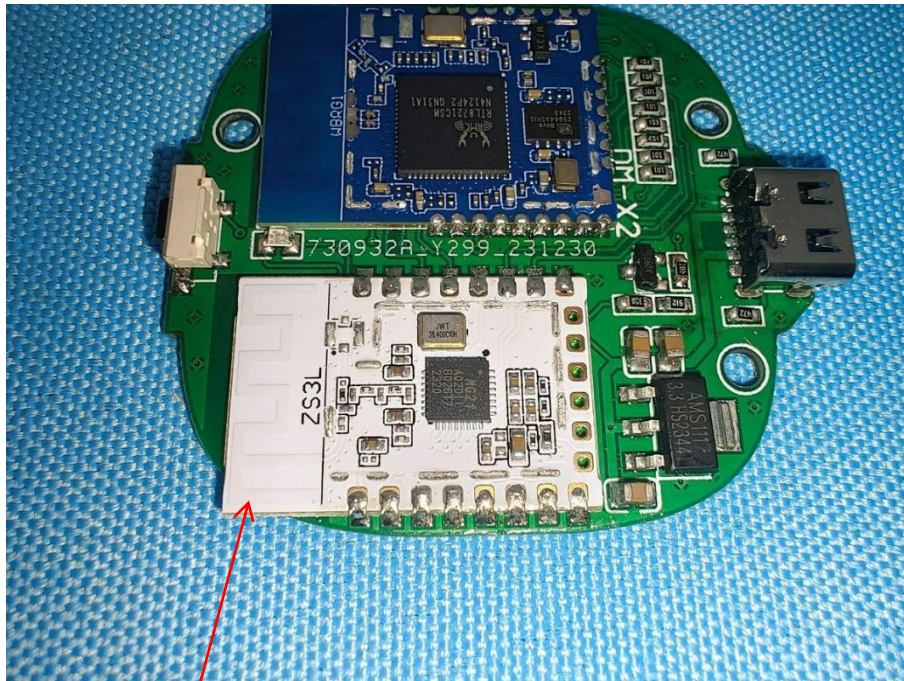
Zigbee ANT:
