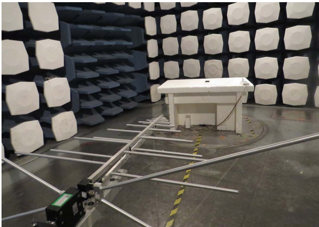
30MHz - 1GHz
