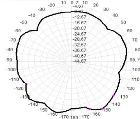
2420.0MHz Total(E2-YZ), Max= -4.88dBi
