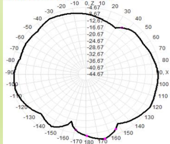
2420.0MHz Total(E1-XZ), Max= -4.67dBi
