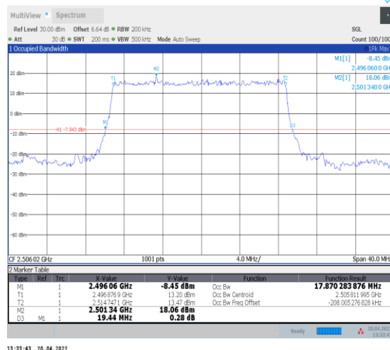
1-N41--30-20-L-2-DFT-PI2BPSK-Outer_Full-50@0-A nt0-17.87-19.440-≤20-PASS
