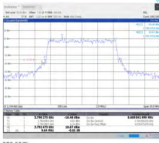
1-N78-3700-3800--30-10-H-8-CP-64QAM-Outer_Full -24@0-Ant0-8.601-9.640-≤10-PASS
