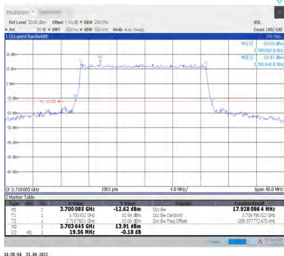
1-N78-3700-3800--30-20-L-3-DFT-16QAM-Outer_Ful I-50@0-Ant0-17.928-19.560-<20-PASS
