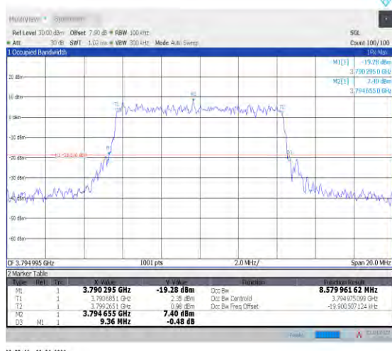
1-N78-3700-3800--30-10-H-9-CP-256QAM-Outer_Fu II-24@0-Ant0-8.58-9.360-≤10-PASS
