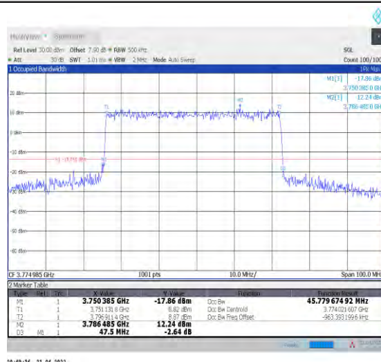
1-N78-3700-3800--30-50-H-3-DFT-16QAM-Outer_Full-128@0-Ant0-45.78-47.500-≤50-PASS
