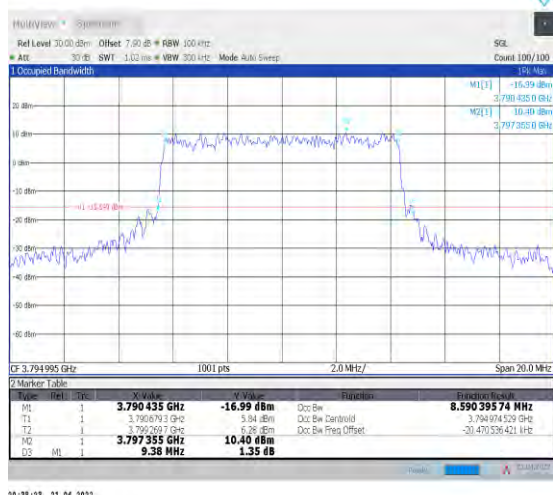
1-N78-3700-3800--30-10-H-7-CP-16QAM-Outer_Full -24@0-Ant0-8.59-9.380-≤10-PASS
