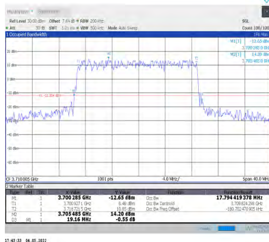
1-N78-3700-3800--30-20-L-4-DFT-64QAM-Outer_Fu II-50@0-Ant0-17.794-19.160-<20-PASS
