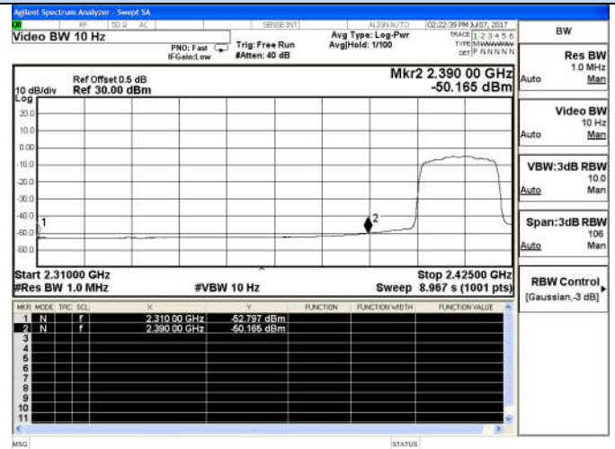
802.11n(HT20)-Low channel(Average)
