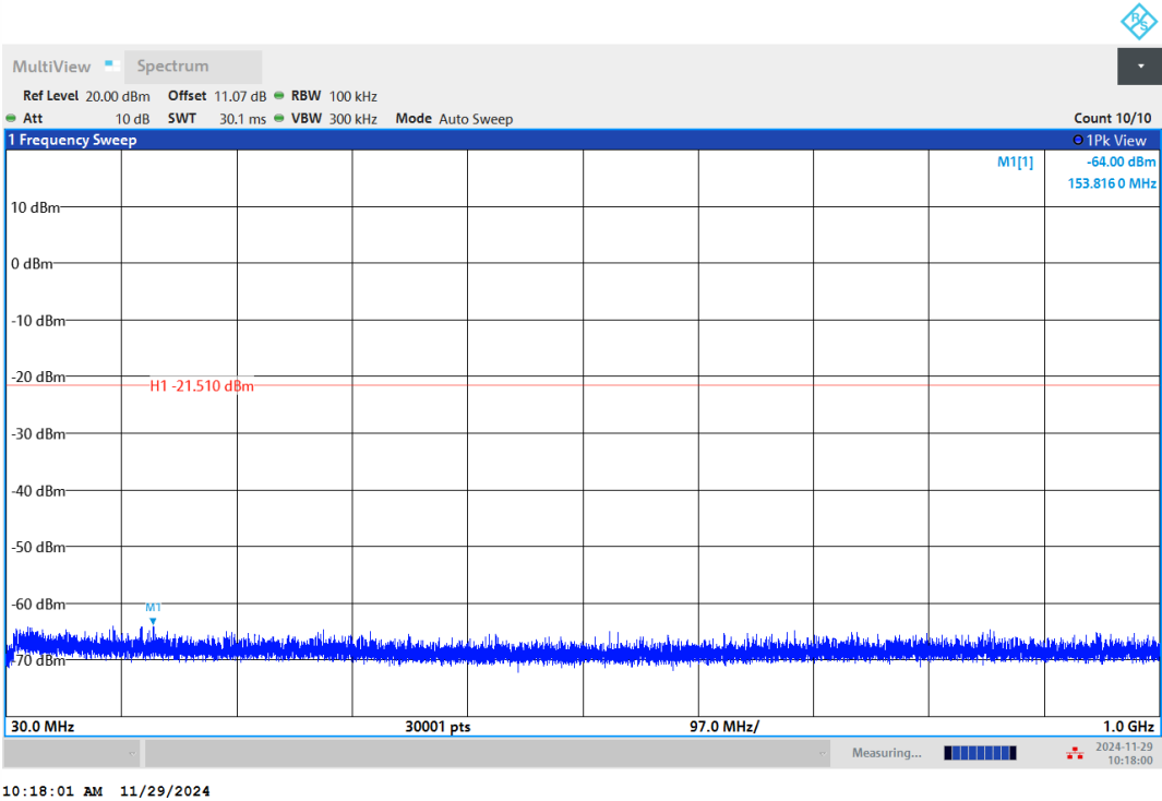
BLE_2M-Ant1-2440-30~1000-PASS
