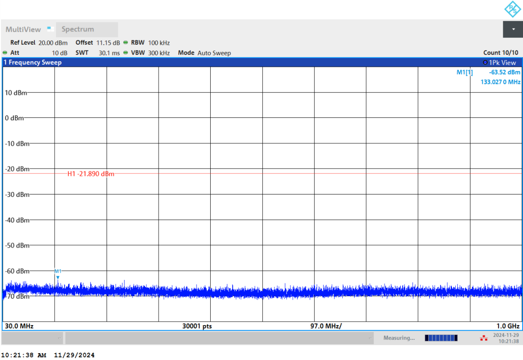
BLE_2M-Ant1-2480-30~1000-PASS
