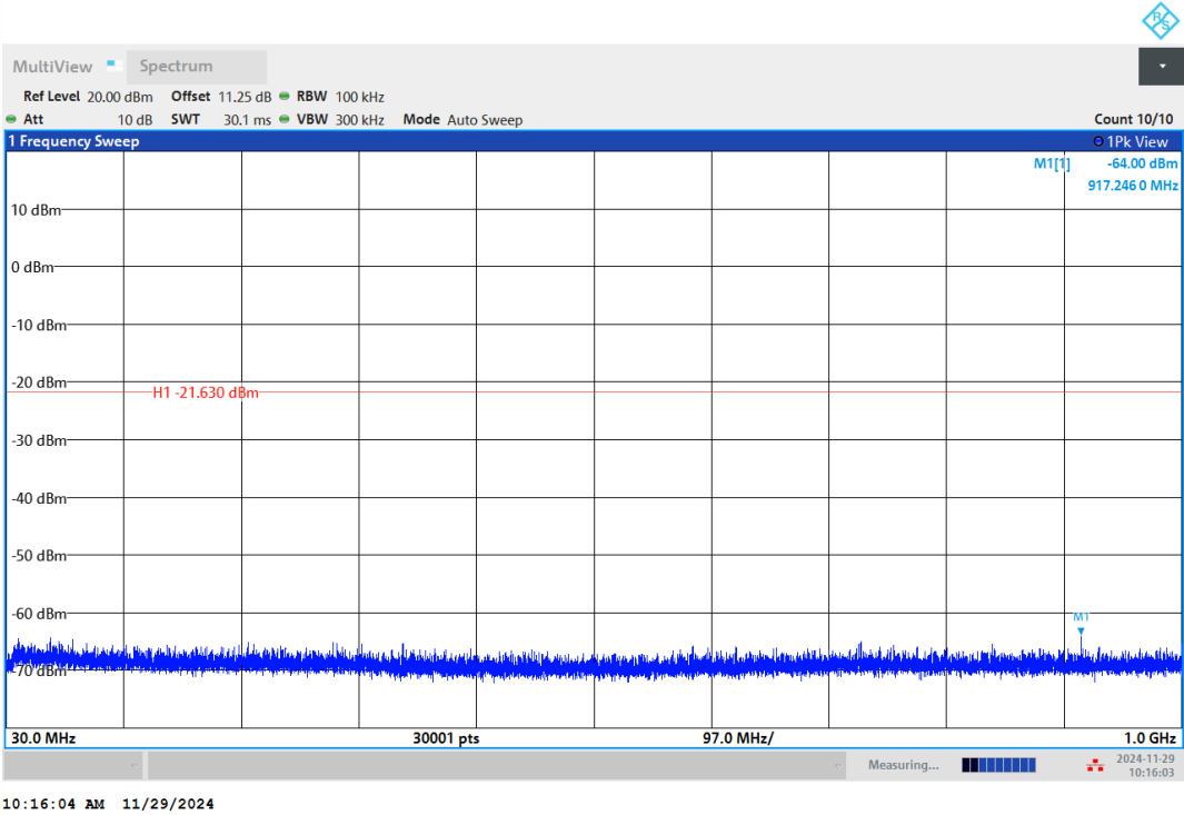
BLE_2M-Ant1-2402-30~1000-PASS
