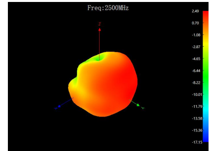
3D 2500MHz
