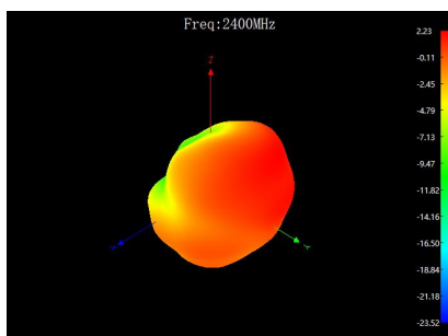
3D 2400MHz
