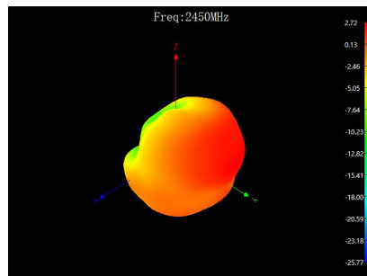
3D 2450MHz
