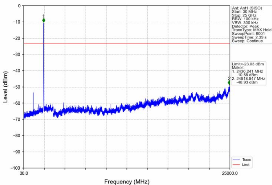
802.11g_MCH_2437MHz_Ant1 (SISO)_NTNV
