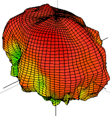
Aux WLAN 5150MHz
