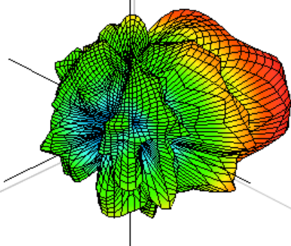
Aux WLAN 2400MHz
