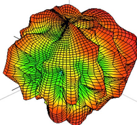
Aux WLAN 2500MHz
