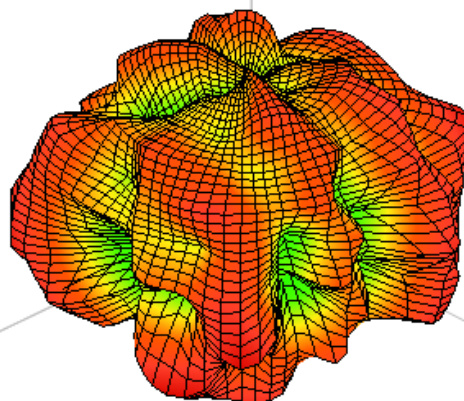
Aux WLAN 2450MHz
