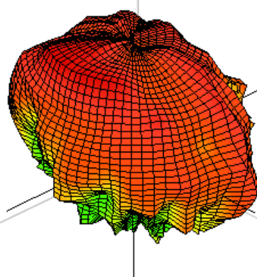
Aux WLAN 5250MHz
