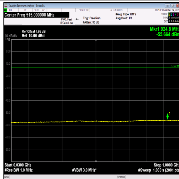
Band4-1312-3-30~1000MHz-PASS
