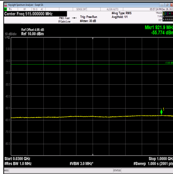
Band2-9538-2-30~1000MHz-PASS
