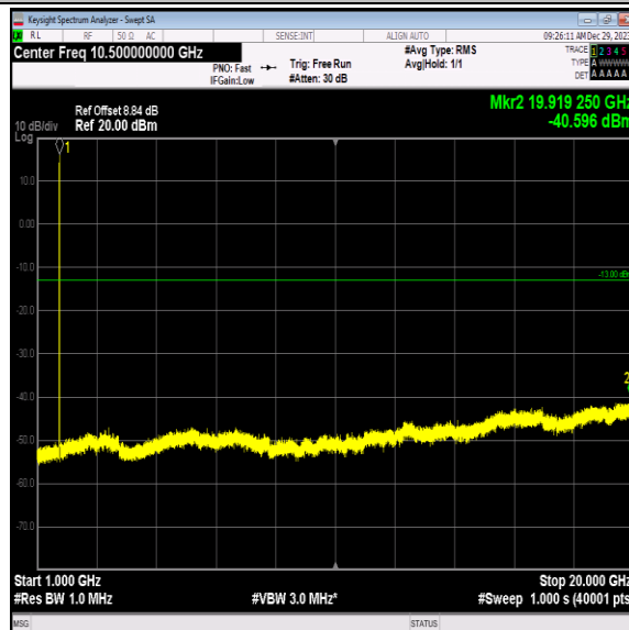
Band4-1312-5-1000~20000MHz-PASS
