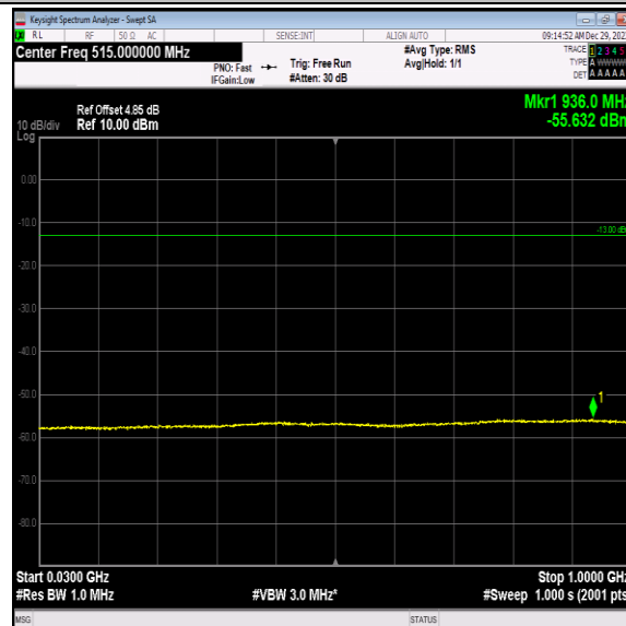
Band4-1312-2-30~1000MHz-PASS
