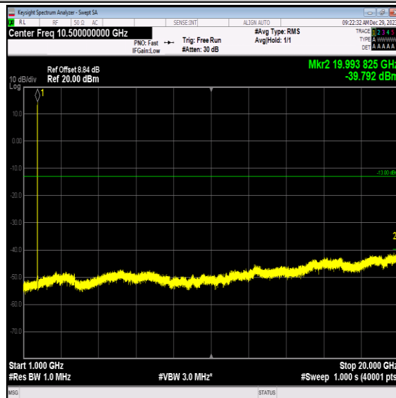
Band4-1312-4-1000~20000MHz-PASS
