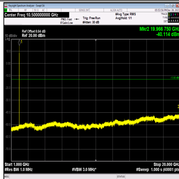
Band2-9538-1-1000~20000MHz-PASS
