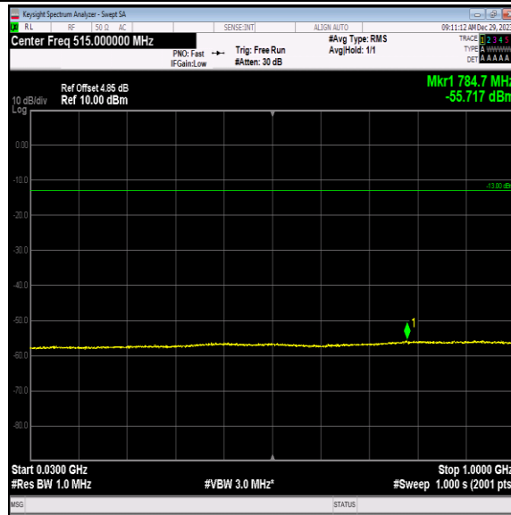
Band4-1312-1-30~1000MHz-PASS
