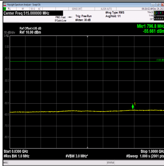
Band4-1312-5-30~1000MHz-PASS
