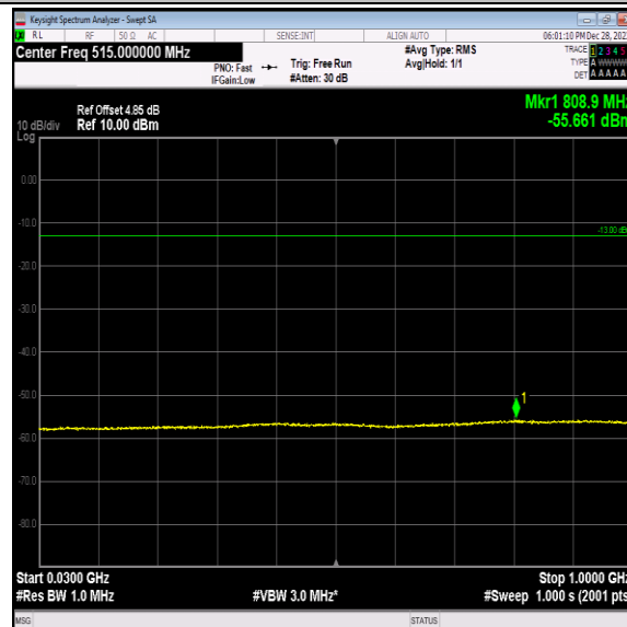
Band2-9538-3-30~1000MHz-PASS
