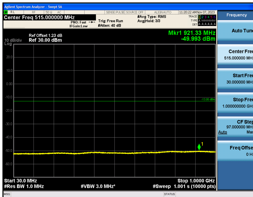
Band4-5MHz-QPSK-20175-1RB#0-Range2:1000~20000MHz
