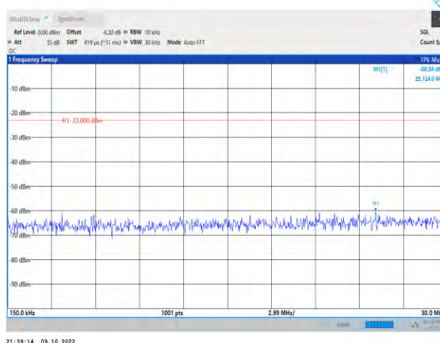
Band66-20MHz-QPSK-132072-1RB#0-Range2:0.15~30MHz
