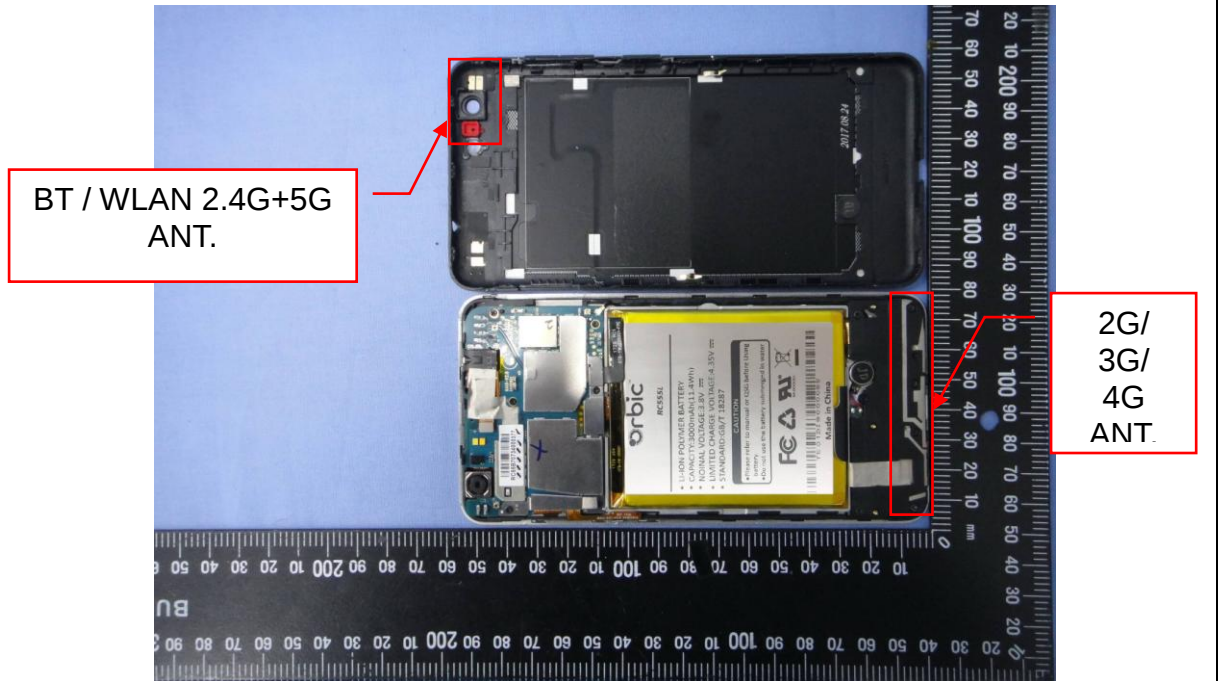
EUT Photo (2)
