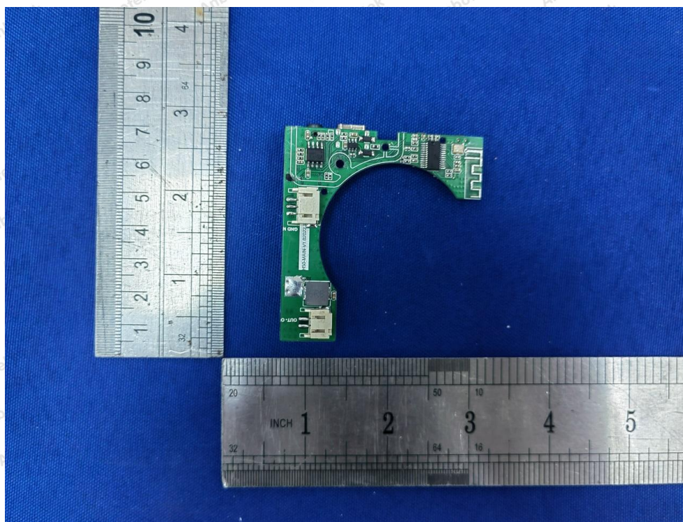
BT ANT
