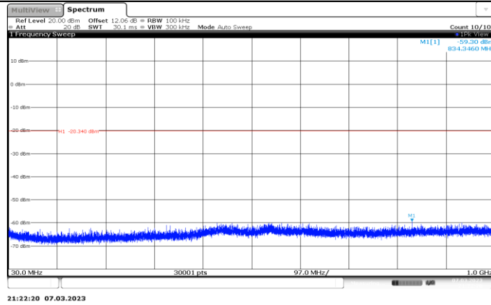
11AX40MIMO_Ant1_2447_30~1000
