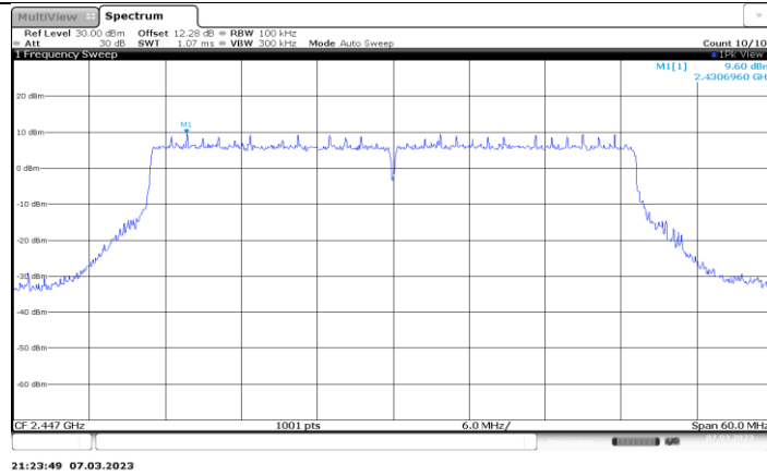
11AX40MIMO_Ant3_2447_0-Reference
