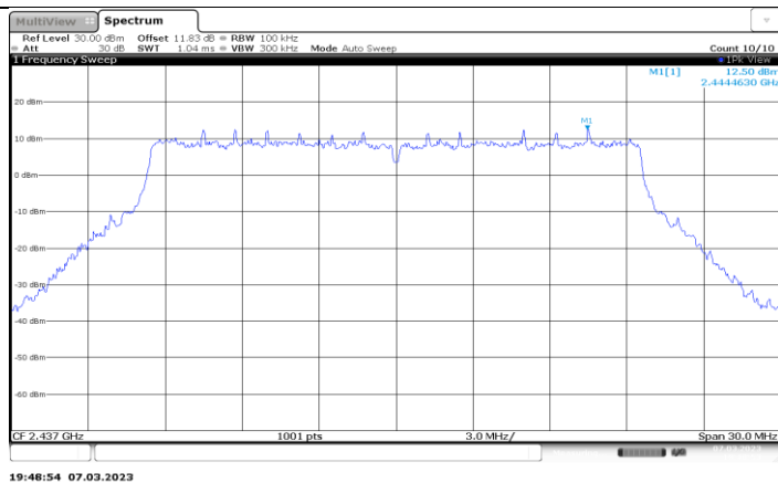
11AX20MIMO_Ant5_2437_0-Reference
