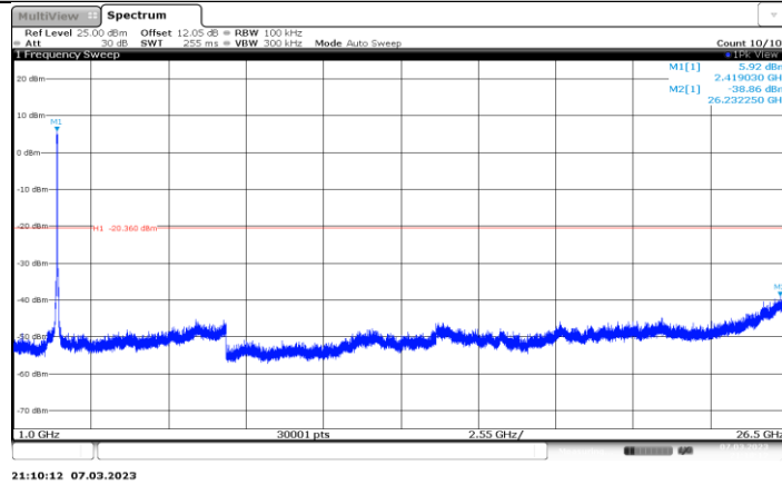
11AX40MIMO_Ant1_2427_1000~26500
