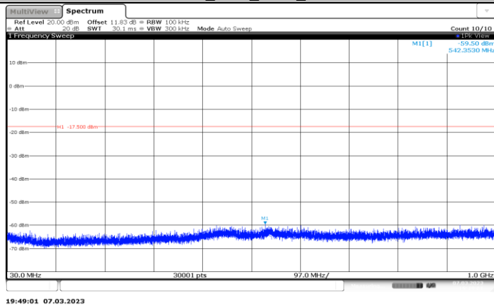
11AX20MIMO_Ant5_2437_30~1000
