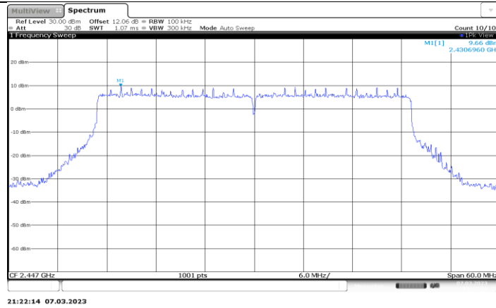
11AX40MIMO_Ant1_2447_0~Reference
