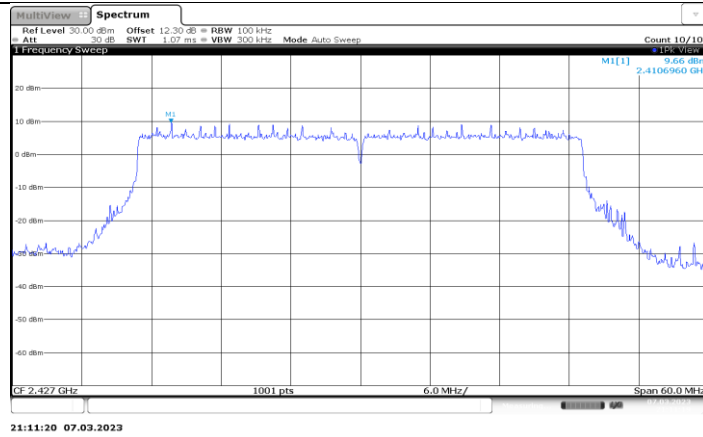
11AX40MIMO_Ant3_2427_0~Reference
