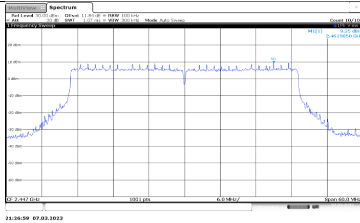
11AX40MIMO_Ant7_2447_0-Reference
