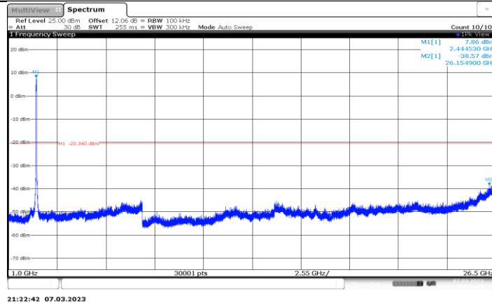
11AX40MIMO_Ant1_2447_1000~26500
