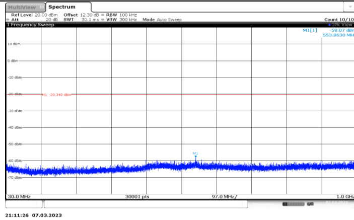
11AX40MIMO_Ant3_2427_30~1000
