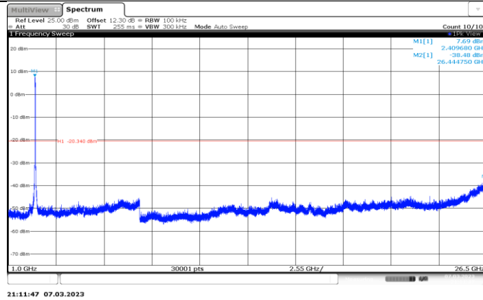
11AX40MIMO_Ant3_2427_1000~26500
