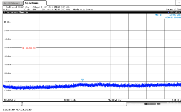
11AX40MIMO_Ant5_2447_30~1000
