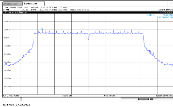
11AX40MIMO_Ant3_2437_0-Reference
