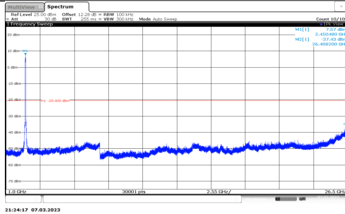
11AX40MIMO_Ant3_2447_1000~26500
