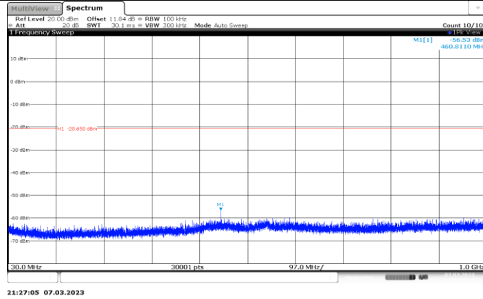
11AX40MIMO_Ant7_2447_30~1000
