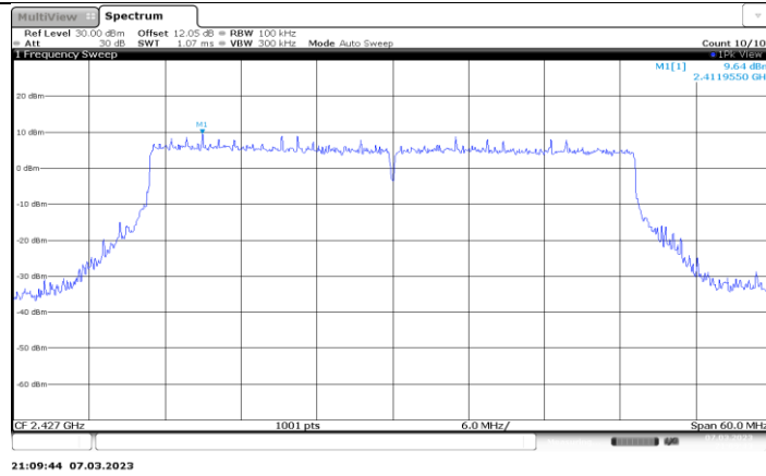
11AX40MIMO_Ant1_2427_0~Reference
