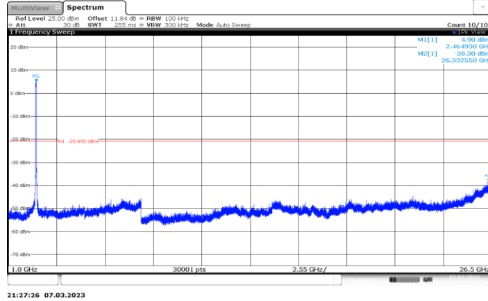
11AX40MIMO_Ant7_2447_1000~26500
