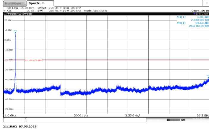
11AX40MIMO_Ant3_2437_1000~26500
