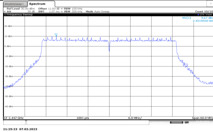
11AX40MIMO_Ant5_2447_0-Reference
