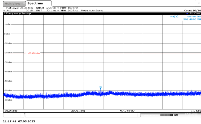
11AX40MIMO_Ant3_2437_30~1000
