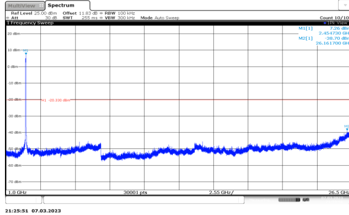
11AX40MIMO_Ant5_2447_1000~26500
