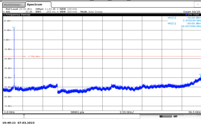
11AX20MIMO_Ant5_2437_1000~26500
