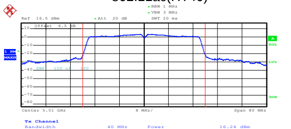
802.11ac(HT40)
