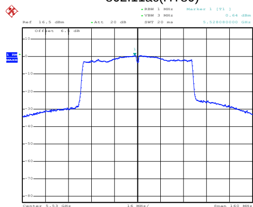
802.11ac(HT80)
