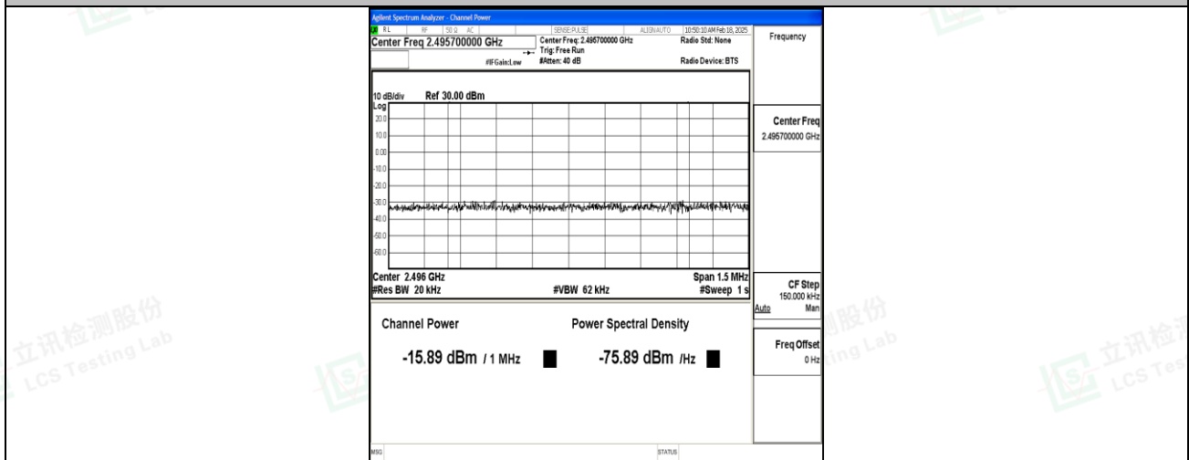
Band7_20MHz_16QAM_20850_100RB#0_Final2
