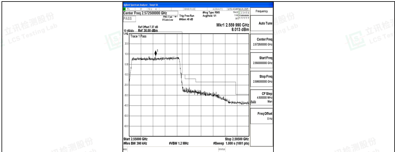
Band7_20MHz_QPSK_21350_100RB#0
