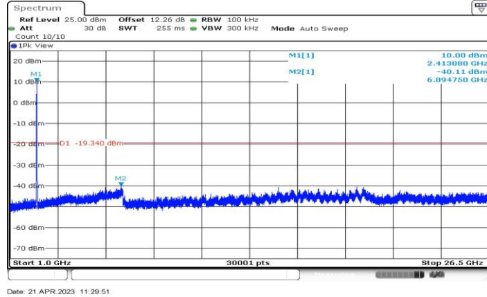
11AX20-CDD_Ant2_2412_1000~26500
