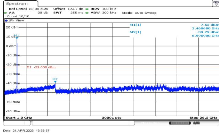
11AX20-CDD_Ant2_2462_1000~26500
