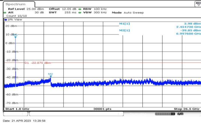
11AX20-CDD_Ant1_2457_1000~26500
