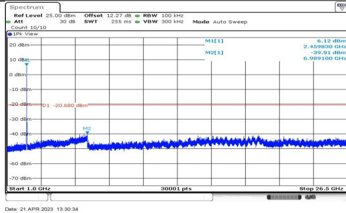
11AX20-CDD_Ant2_2457_1000~26500
