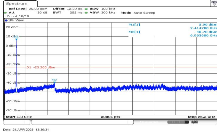
11AX40-CDD_Ant2_2422_1000~26500
