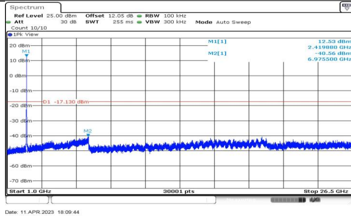
11AX20-CDD_Ant1_2417_1000~26500
