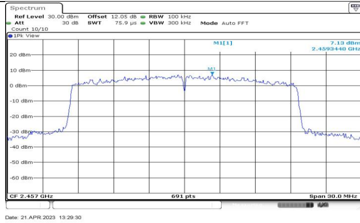
11AX20-CDD_Ant1_2457_0~Reference
