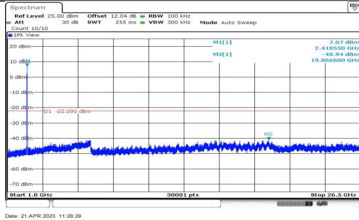
11AX20-CDD_Ant1_2412_1000~26500
