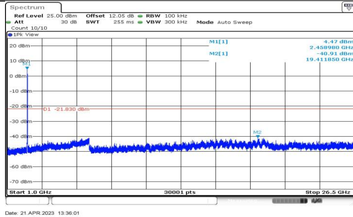
11AX20-CDD_Ant1_2462_1000~26500
