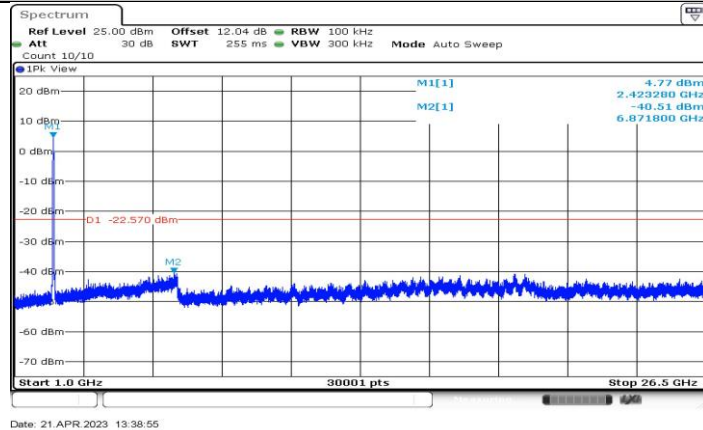
11AX40-CDD_Ant1_2422_1000~26500
