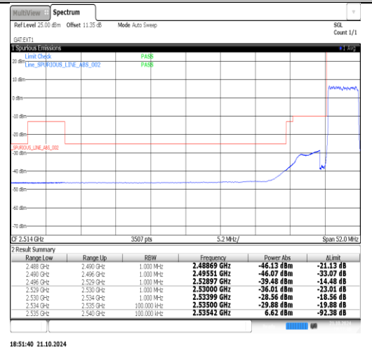
41(2535-2655)-5MHz-QPSK-41215-1RB#0-PASS
