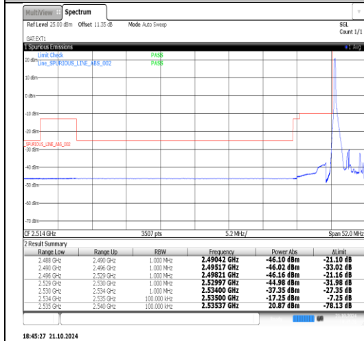
41(2535-2655)-5MHz-QPSK-40065-1RB#24-PASS
