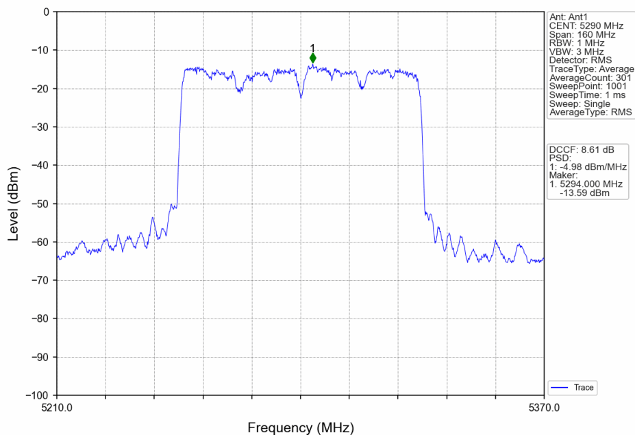
802.11ax(HEW80)_MCH_5290MHz_RU996_Left_Ant1_NTNV
