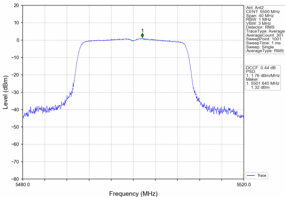
802.11ax(HEW20)_LCH_5500MHz_RU242_Left_Ant2_NTNV
