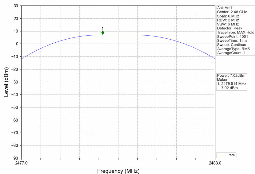
2M_HCH_2480MHz_DataRate=_Ant1_NTNV
