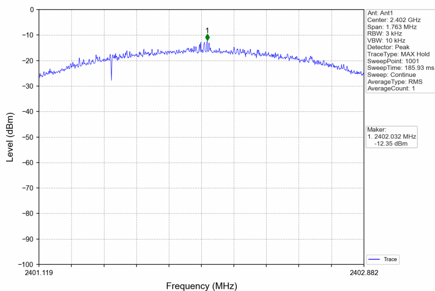
2M_LCH_2402MHz_DataRate=_Ant1_NTNV
