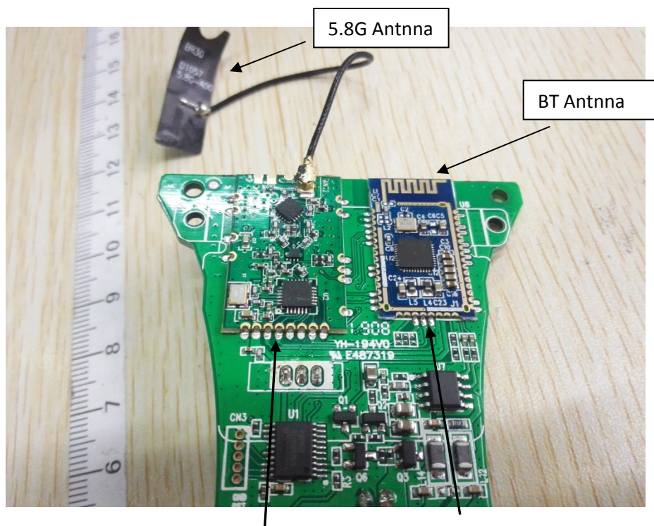
5.8G Module BT Module
