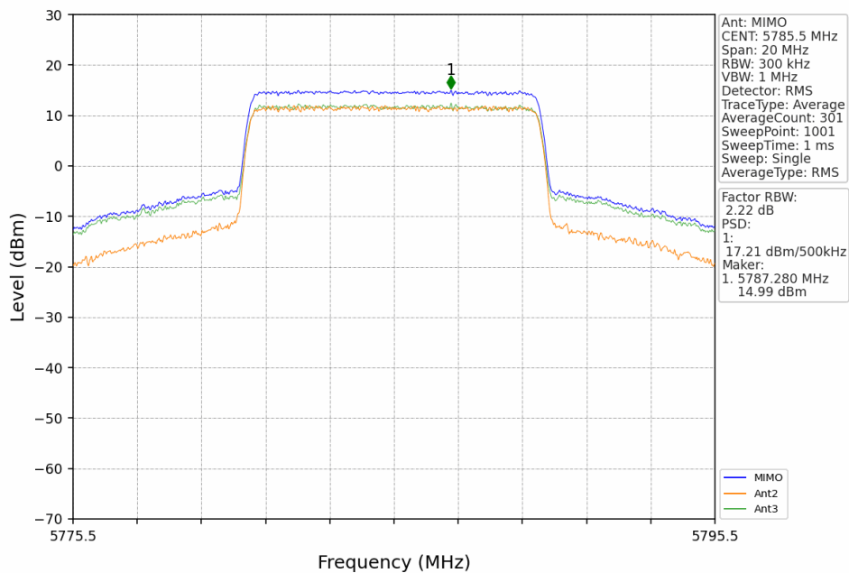
10M_MCH_5785.5MHz_MIMO_NTNV
