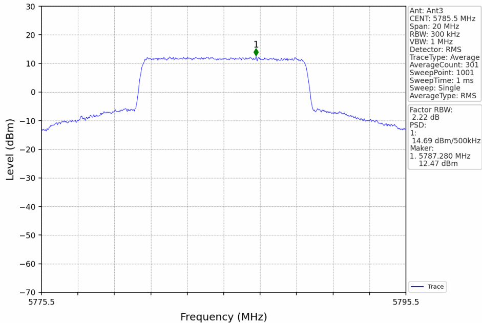
10M_MCH_5785.5MHz_MIMO_NTNV
