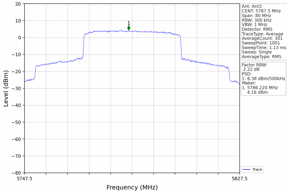
40M_MCH_5787.5MHz_MIMO_NTNV
