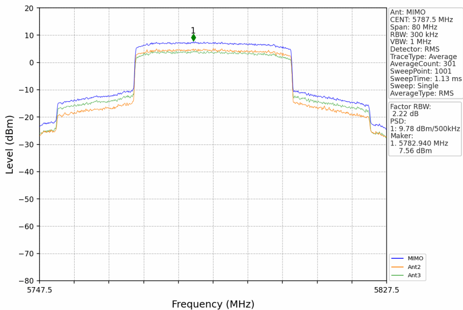
40M_MCH_5787.5MHz_MIMO_NTNV
