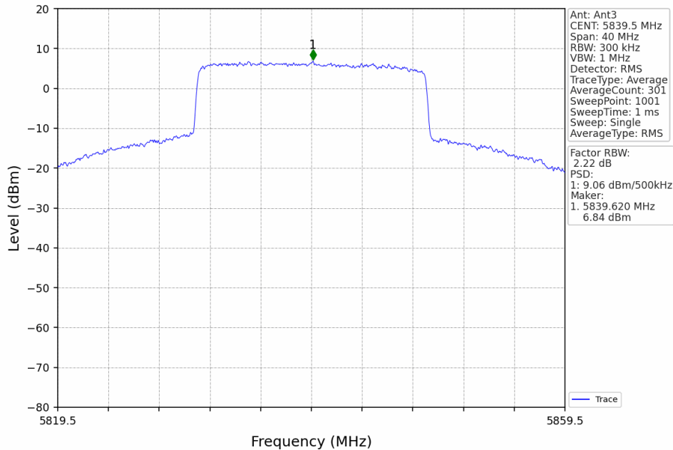
20M_HCH_5839.5MHz_MIMO_NTNV
