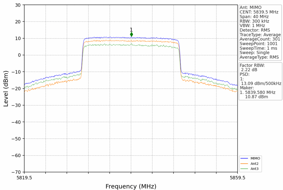
20M_HCH_5839.5MHz_MIMO_NTNV
