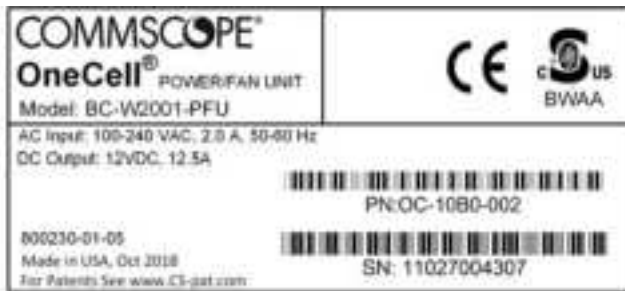
Figure 3-1. Fan label
