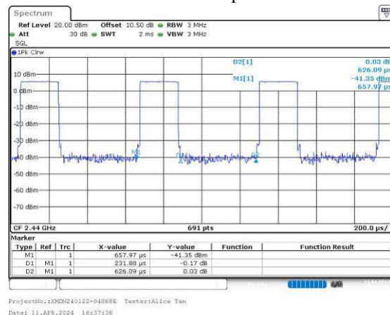
BLE 2Mbps
