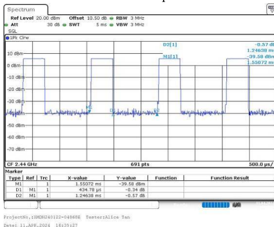
BLE 1Mbps
