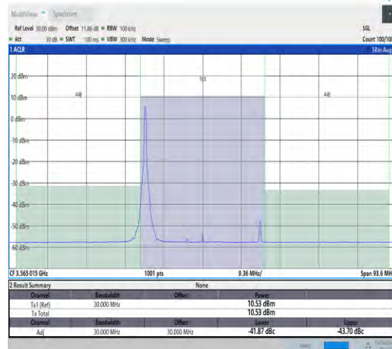
NTNV_N48_30_30_L_TID2_#1_-30_30
