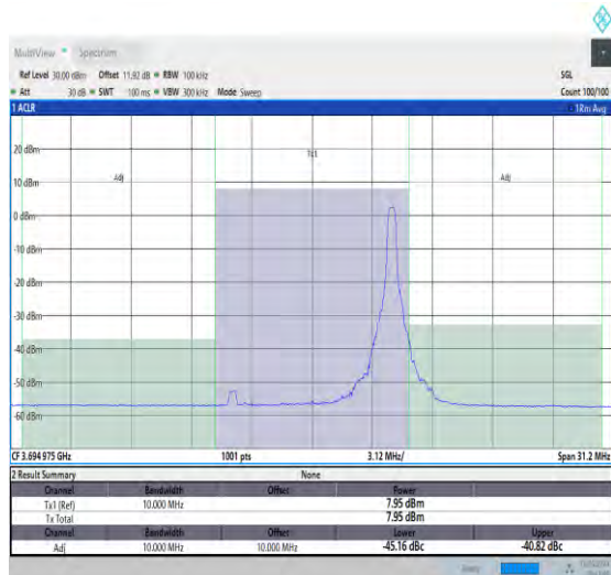
NTNV_N48_30_10_H_TID18_#1_-10_10
