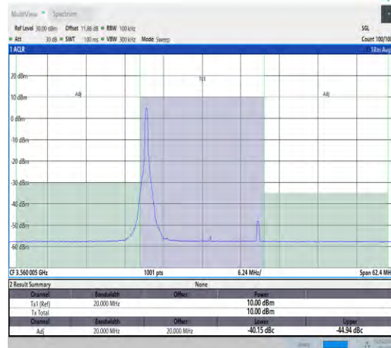
NTNV_N48_30_20_L_TID2_#1_-20_20
