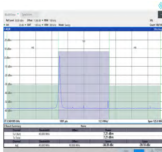
NTNV_N48_30_40_L_TID17_#1_-40_40
