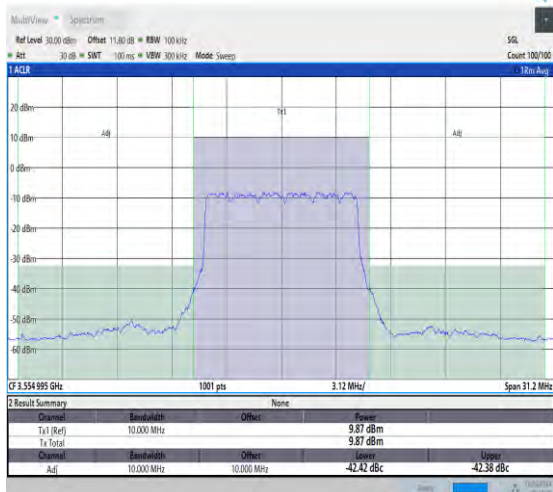
NTNV_N48_30_10_L_TID1_#1_-10_10
