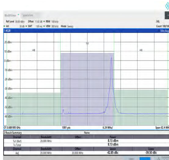
NTNV_N48_30_20_H_TID18_#1_-20_20
