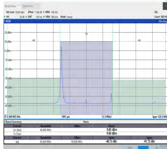
NTNV_N48_30_40_L_TID2_#1_-40_40
