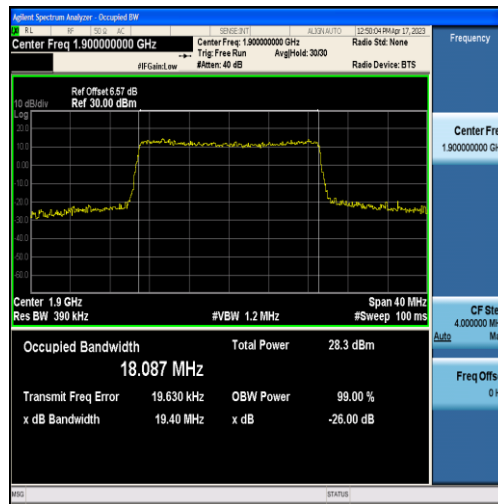
Band2-20MHz-16QAM-19100-100RB#0-18.087
