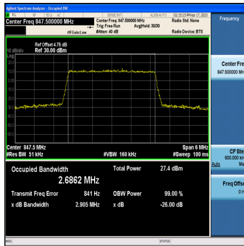
Band5-3MHz-QPSK-20635-15RB#0-2.6862
