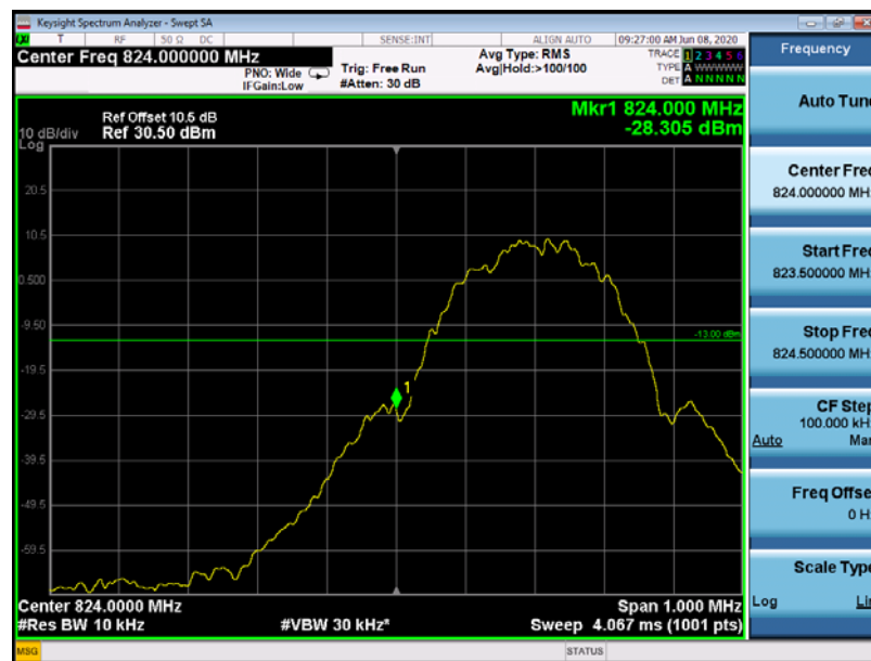
(Plot A: GPRS 850 Channel = 128)
