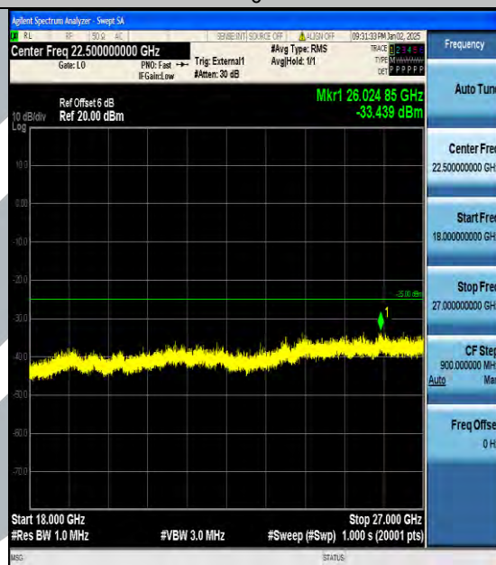
Band38_15MHz_QPSK_38000_1RB#0_18000~27000_18000~27000
