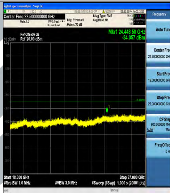
Band38_15MHz_16QAM_38175_1RB#0_18000~27000_18000~27000
