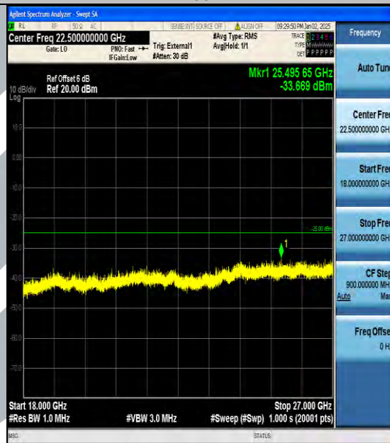
Band38_15MHz_16QAM_37825_1RB#0_18000~27000_18000~27000
