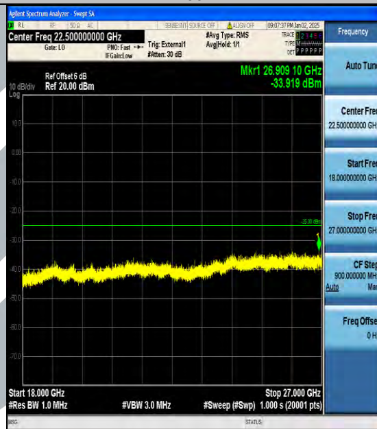
Band38_10MHz_16QAM_38200_1RB#0_18000~27000_18000~27000
