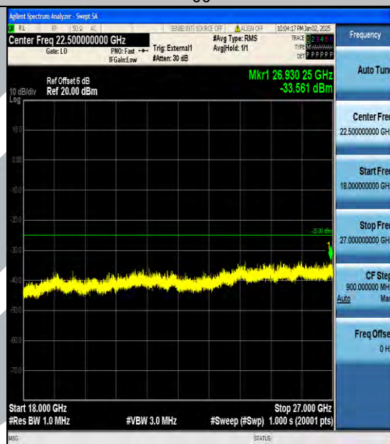
Band38_20MHz_16QAM_38150_1RB#0_18000~27000_18000~27000
