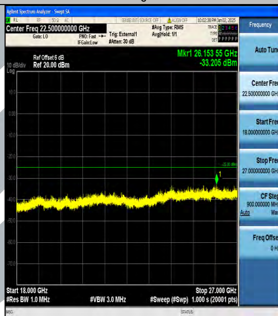
Band38_20MHz_QPSK_38150_1RB#0_18000~27000_18000~27000
