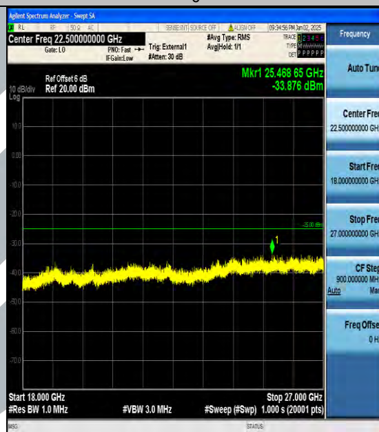
Band38_15MHz_QPSK_38175_1RB#0_18000~27000_18000~27000
