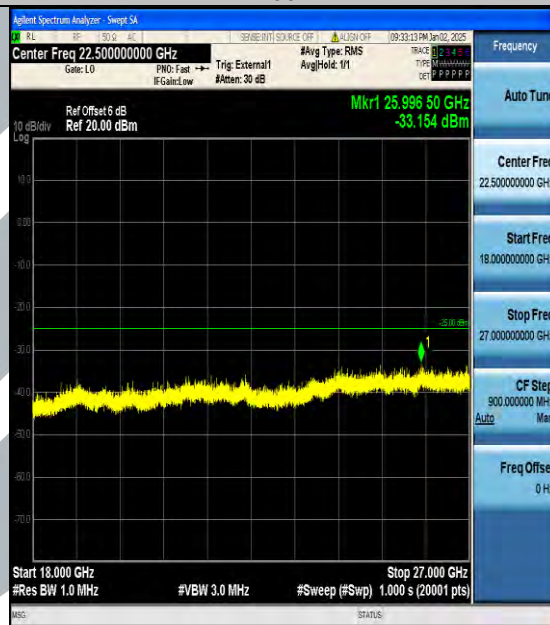
Band38_15MHz_16QAM_38000_1RB#0_18000~27000_18000~27000
