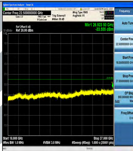
Band38_20MHz_16QAM_38000_1RB#0_18000~27000_18000~27000
