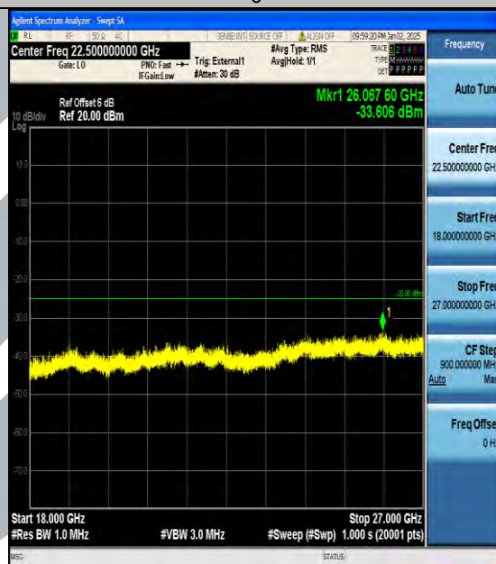
Band38_20MHz_QPSK_38000_1RB#0_18000~27000_18000~27000
