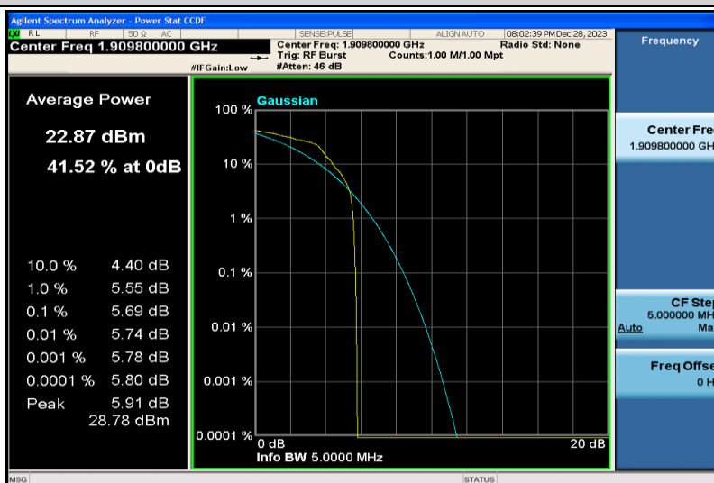
EGPRS1900-810
