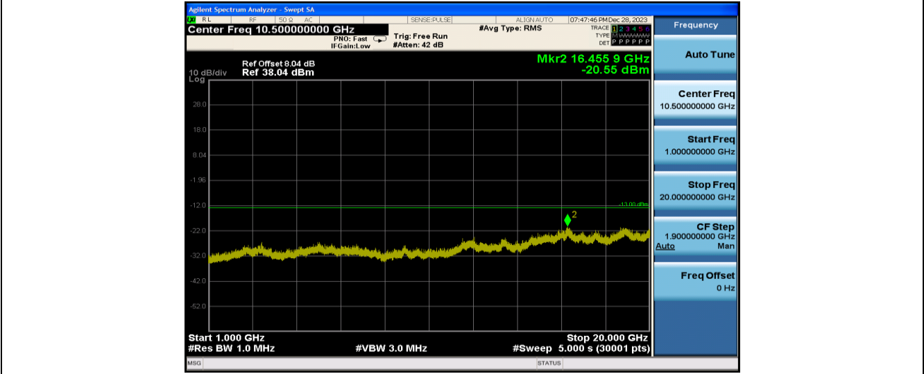
GPRS1900-810-1000~20000
