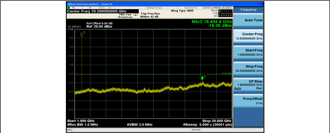
GPRS1900-661-1000~20000
