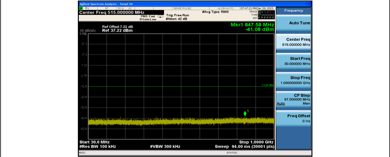
GPRS1900-810-30~1000
