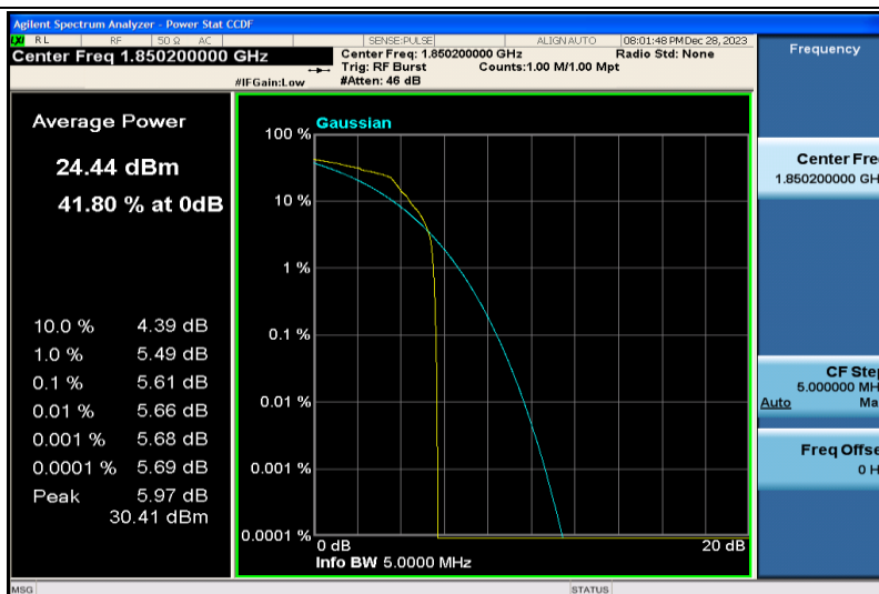
EGPRS1900-512
