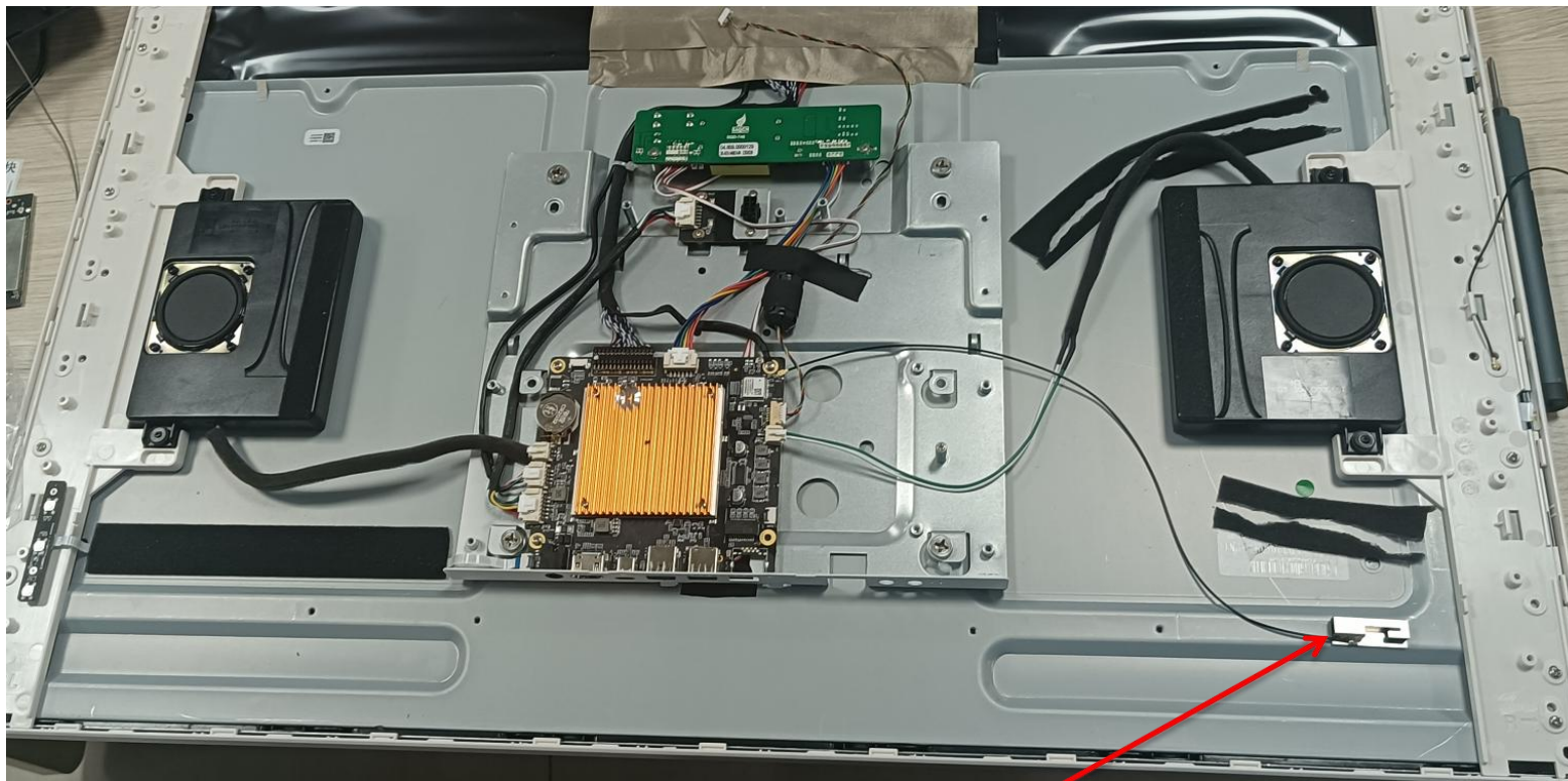
WIFI1天线
