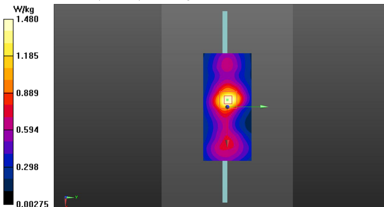
Fig. 23 NR n77 (Part 27O) Body
