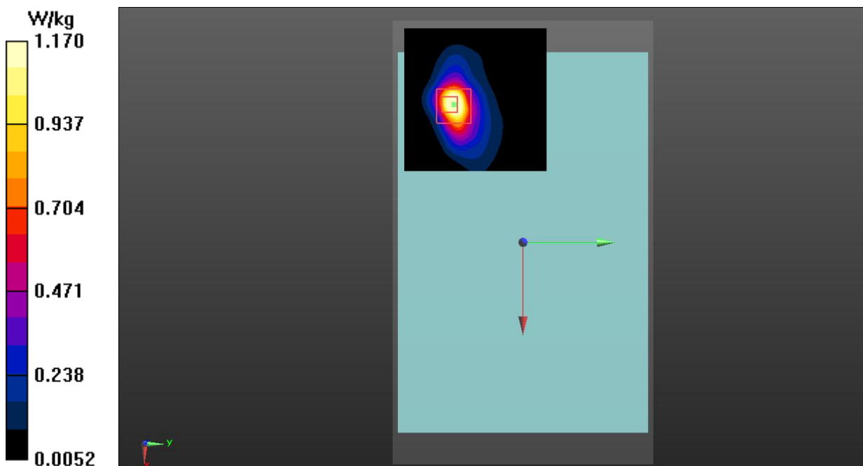
Fig. 25 WLAN 2.4GHz Body
