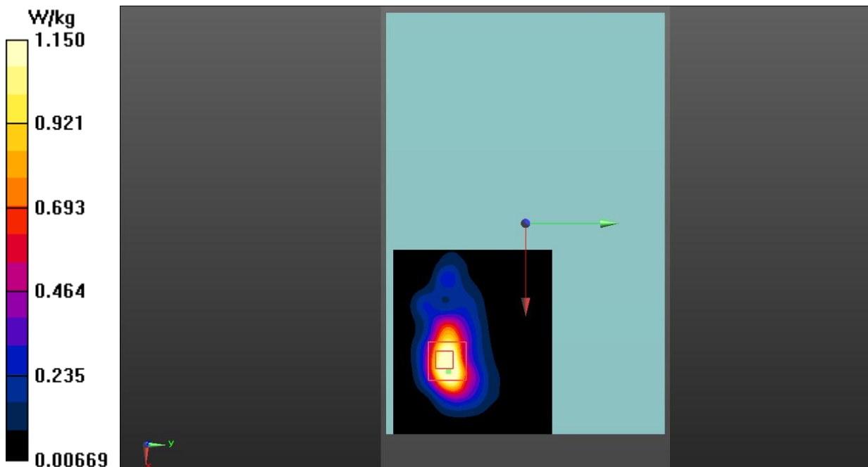
Fig. 17 NR n2 Body
