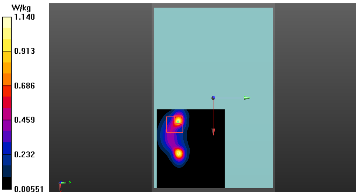
Fig. 1 GSM850 Body
