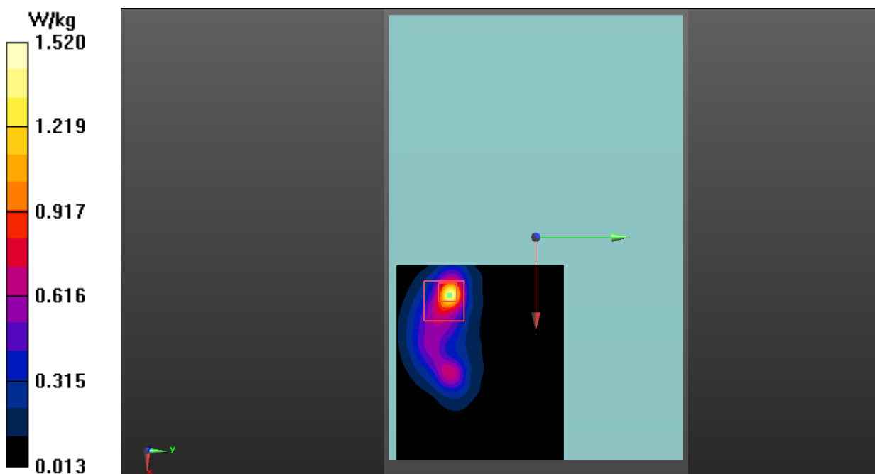
Fig. 21 NR n71 Body
