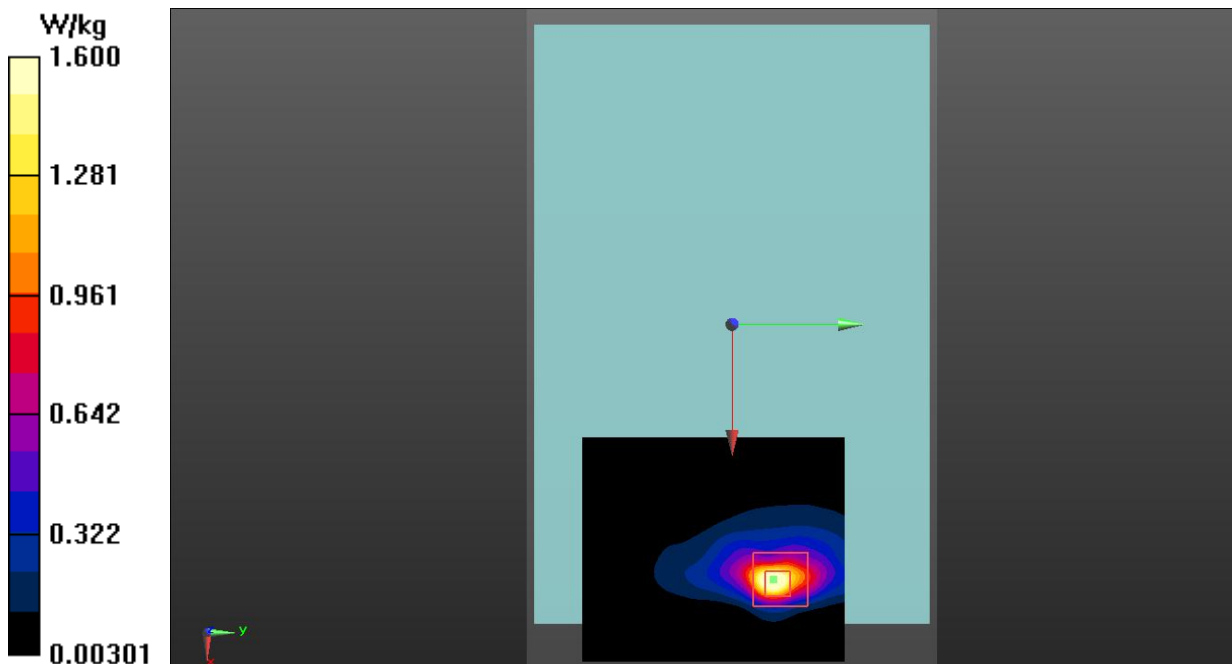
Fig. 19 NR n41 Body
