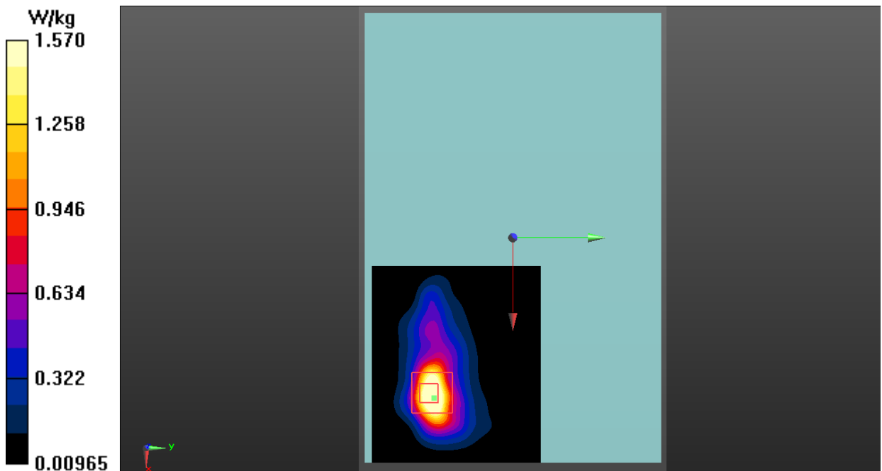
Fig. 2 GSM1900 Body
