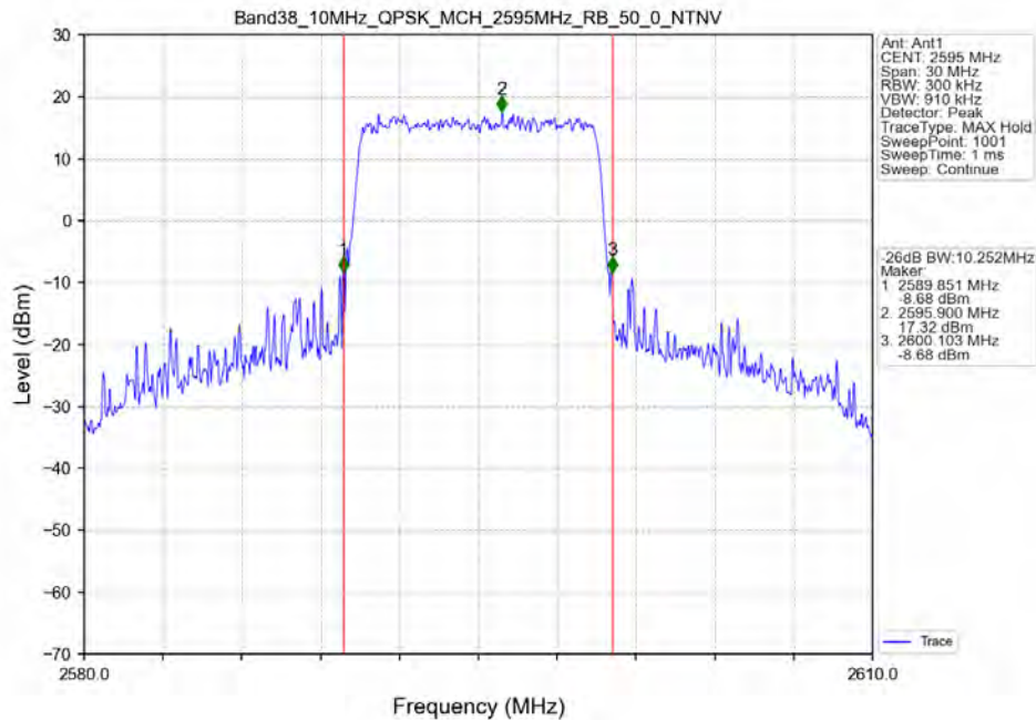
Band38_10MHz_QPSK_MCH_2595MHz_RB_50_0_NTNV
