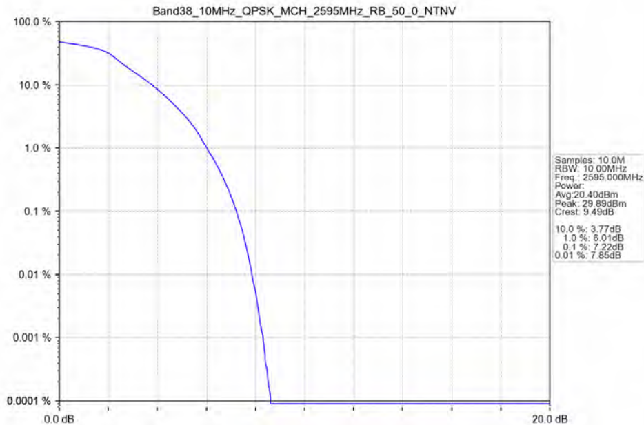
Band38_10MHz_QPSK_MCH_2595MHz_RB_50_0_NTNV
