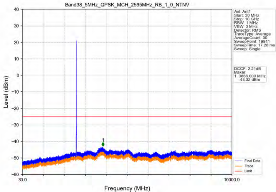
Band38_5MHz_QPSK_MCH_2595MHz_RB_1_0_NTNV
