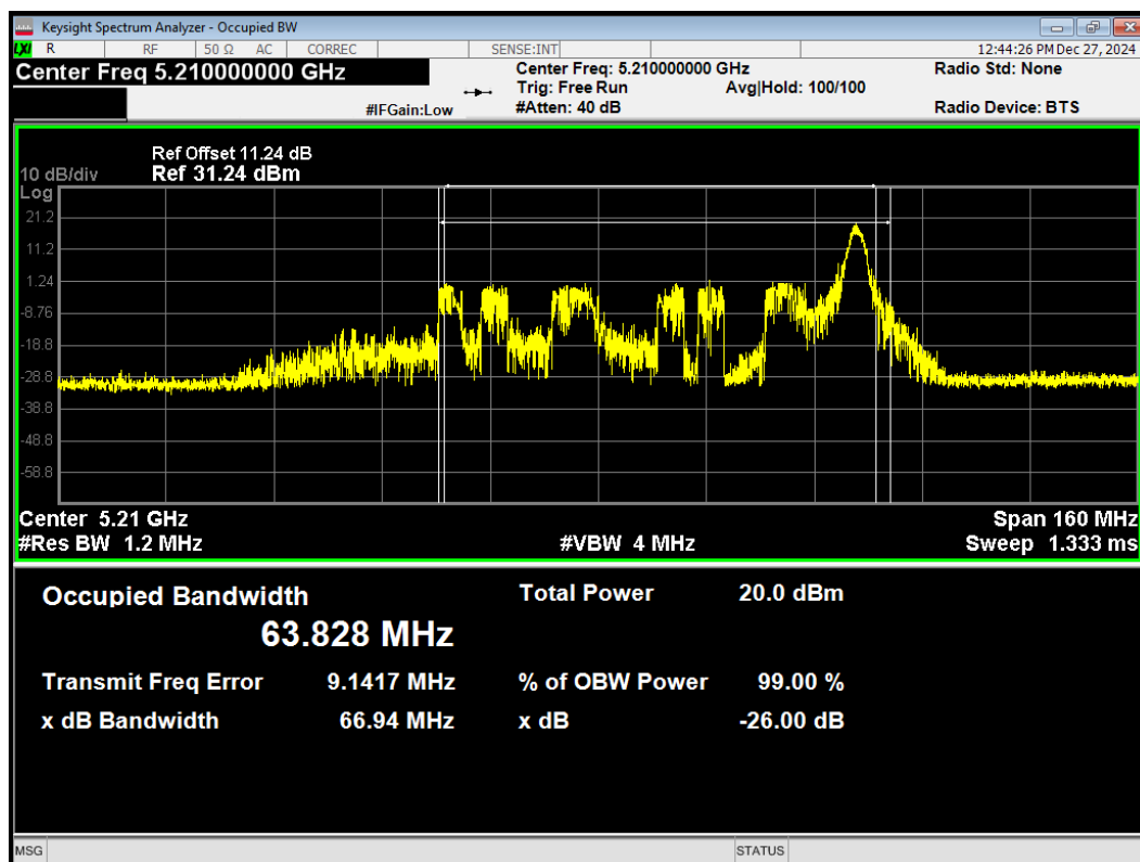
OBW 802.11ax HE80 26-Tones 5210MHz
