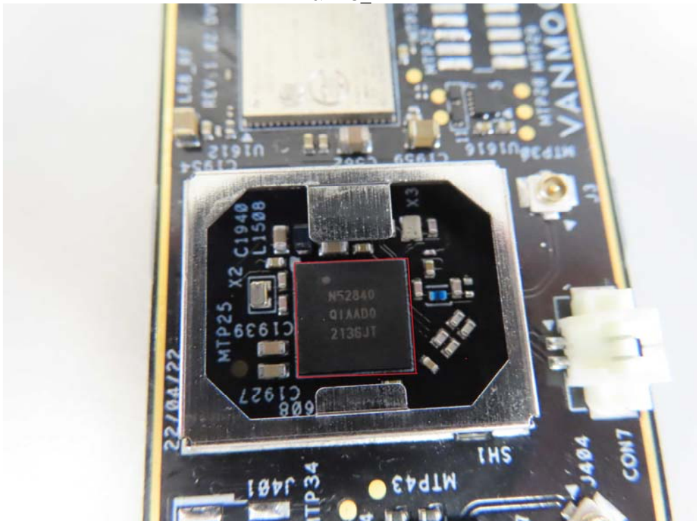
GPS&WWAN_Module
