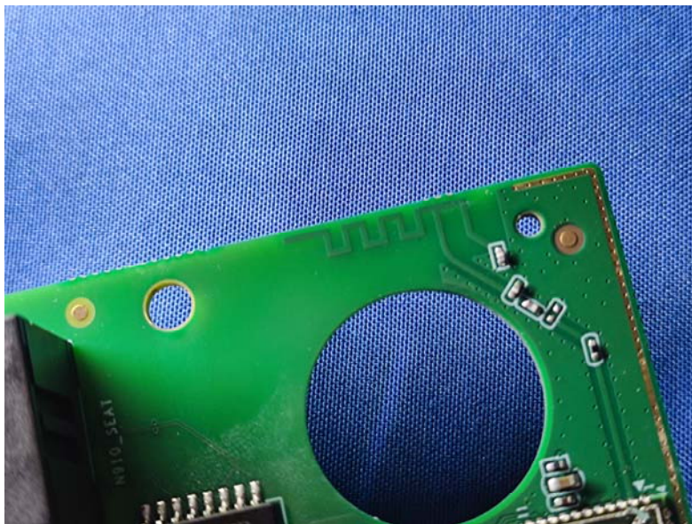
BT&WIFI Antenna
