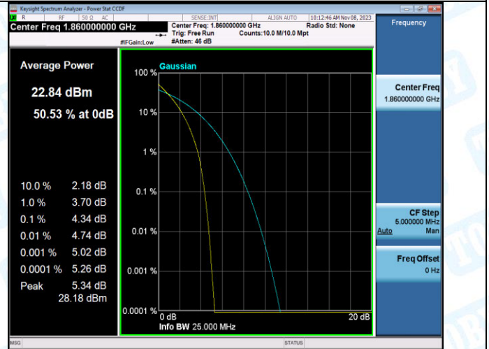
Band2-20MHz-QPSK-18700-100RB#0-PASS
