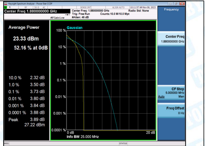
Band2-20MHz-QPSK-18900-1RB#0-PASS
