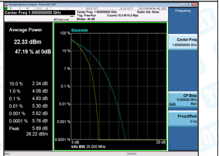
Band2-20MHz-QPSK-19100-100RB#0-PASS
