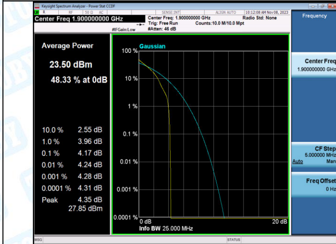
Band2-20MHz-QPSK-19000-1RB#0-PASS
