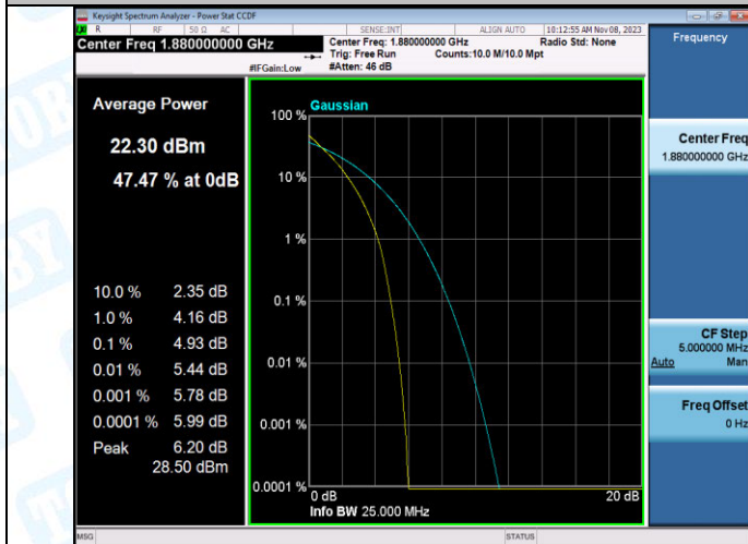
Band2-20MHz-QPSK-18900-100RB#0-PASS
