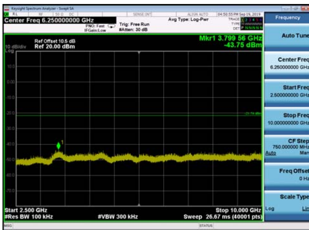
,Plot 4,2500MHz~10000MHz-802.11g ,2437MHz,Ant0
