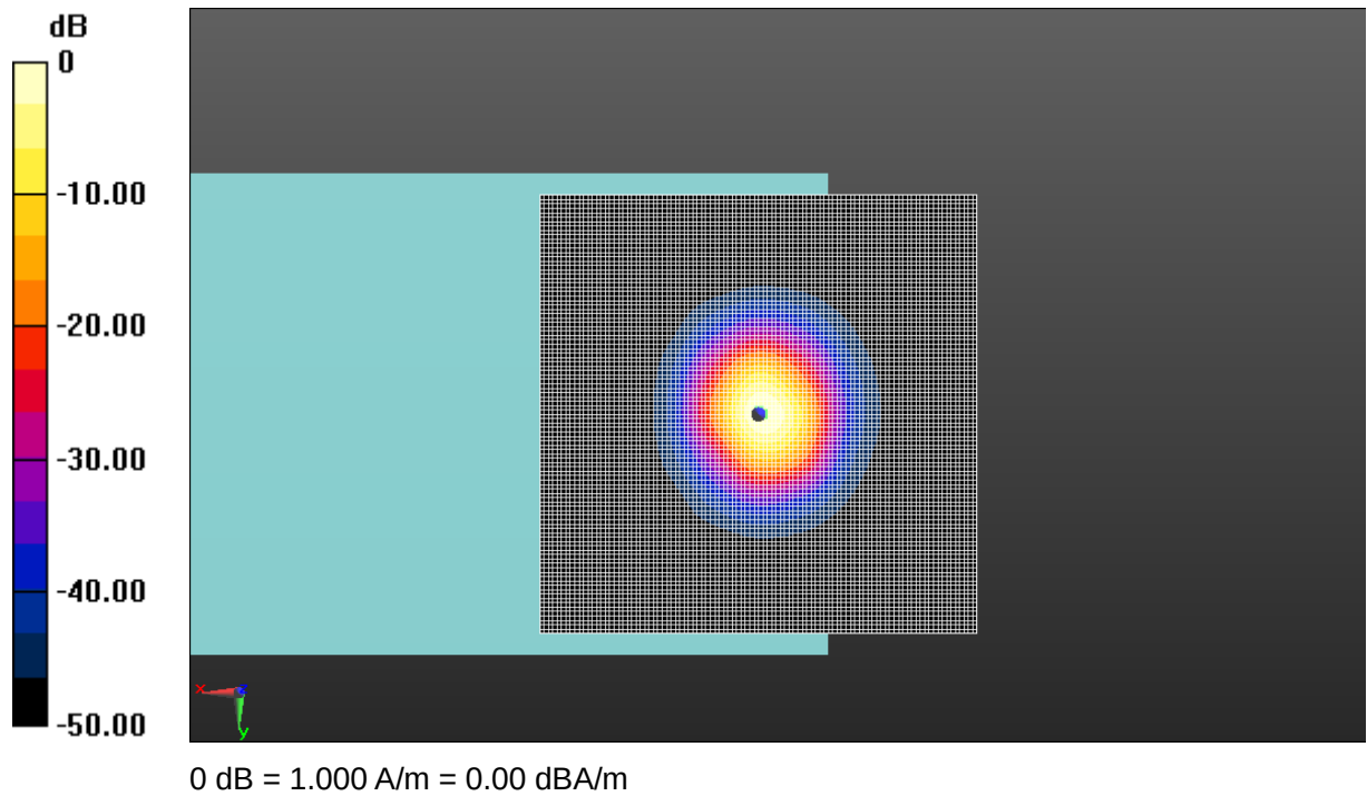
Fig A.9 T-Coil WCDMA B5
