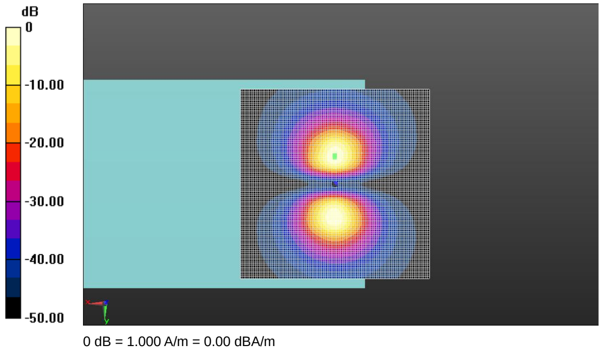
Fig A.8 T-Coil WCDMA B4
