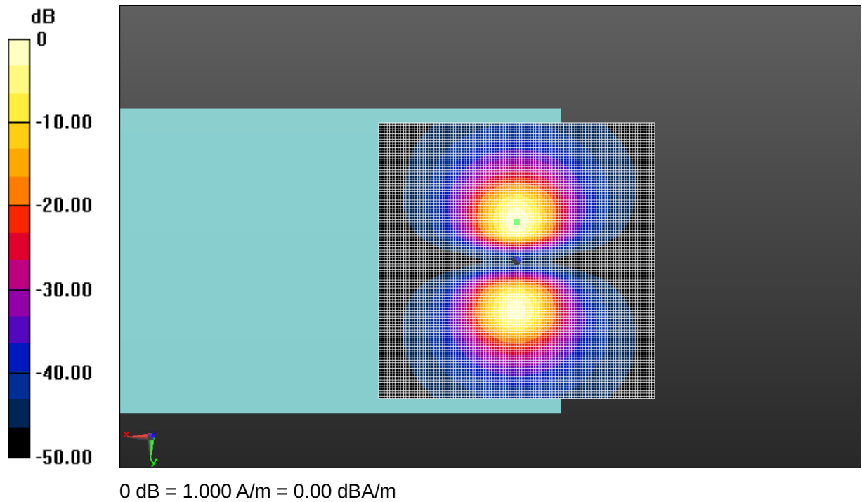
Fig A.10 T-Coil WCDMA B5
