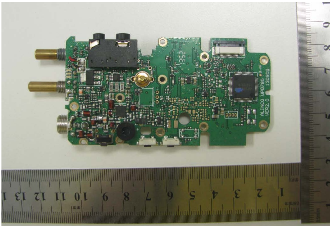
3. Mainboard
