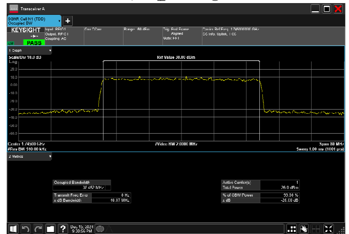
n66_40MHz_15kHz_1745MHz_CP-OFDM QPSK_RB216@0
