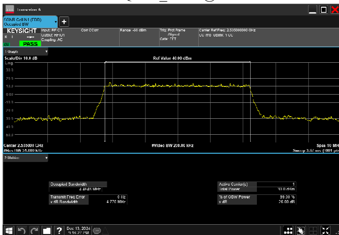
n7_5MHz_15kHz_2535MHz_DFT-s-OFDM QPSK_RB25@0
