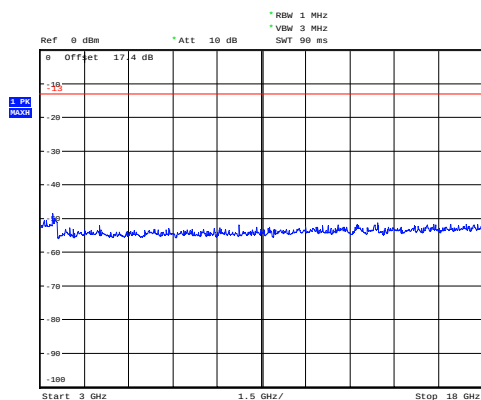
WCDMA Band IV CH-Low 3GHz~18GHz
