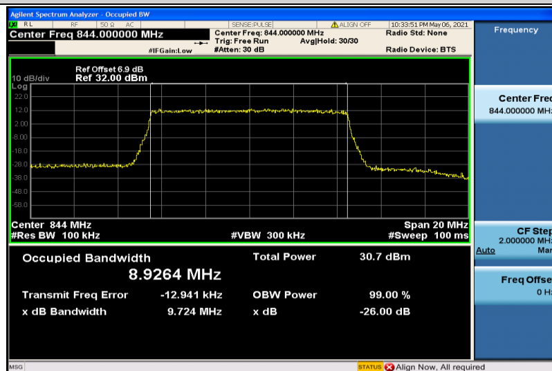
Band5-10MHz-QPSK-20600-50RB#0-8.9264
