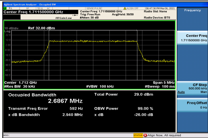
Band4-3MHz-16QAM-19965-15RB#0-2.6867
