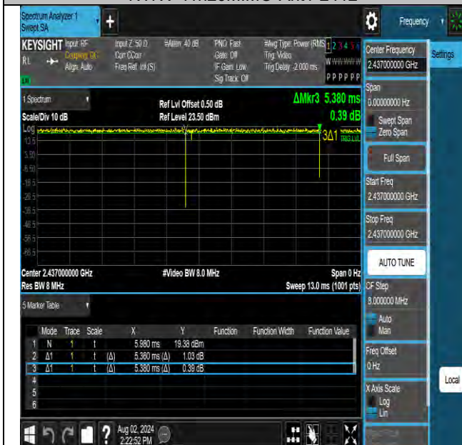
NTNV-11n20MIMO-Ant1-2437
