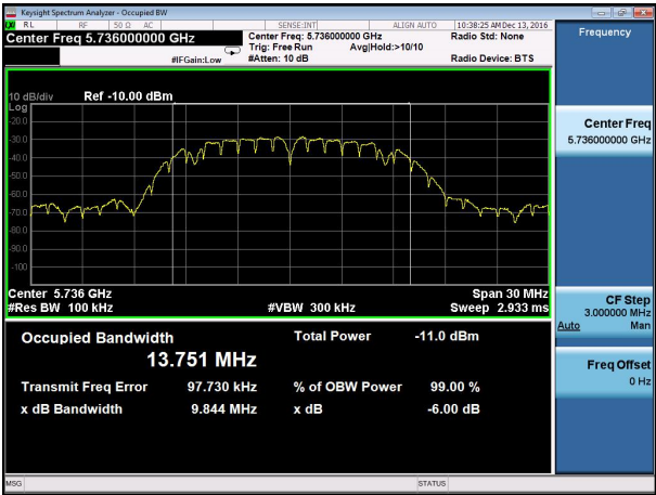
5736MHz-ANTB
